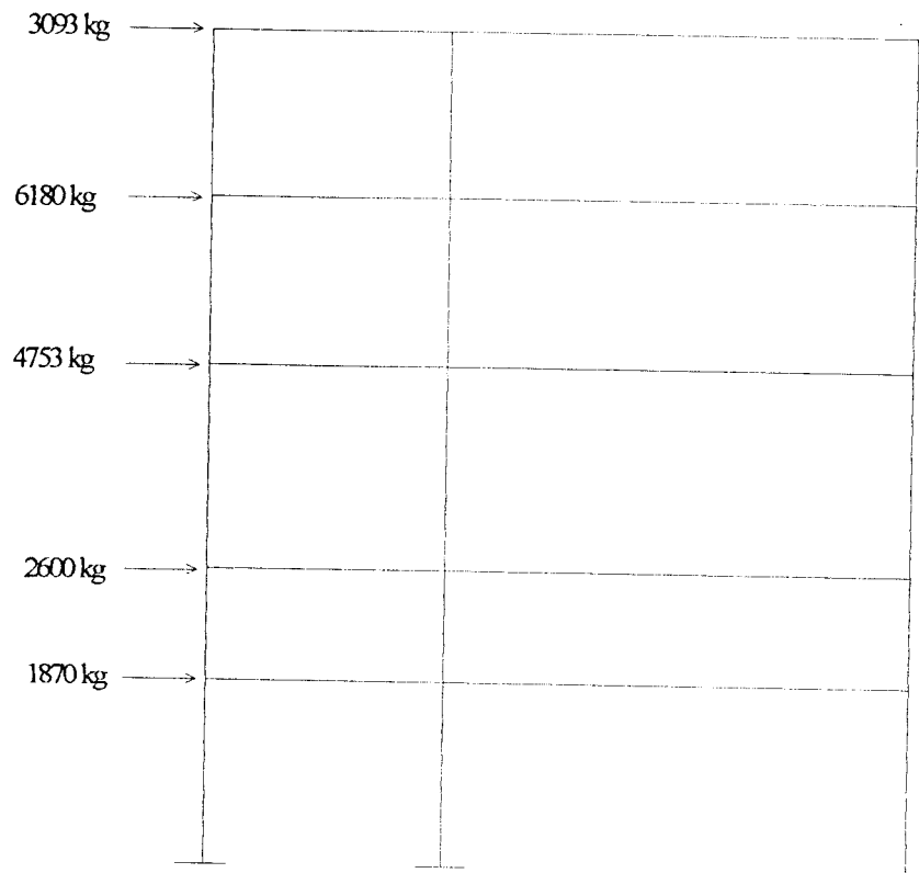
Gambar 4.9 Distribusi beban gempa untuk portal arah y
