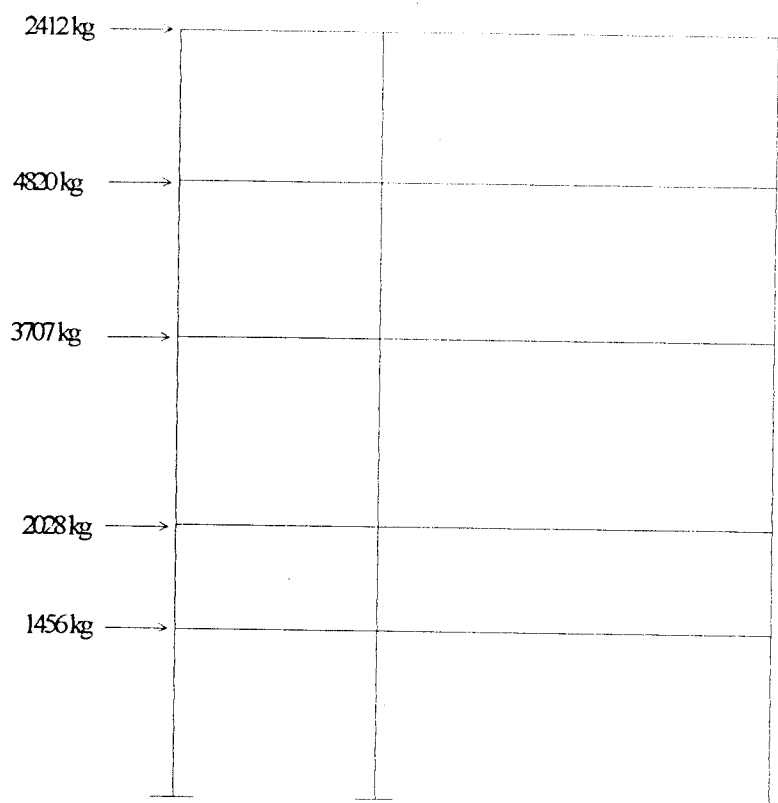
Gambar 4.11 Distribusi beban gempa untuk portal arah y
