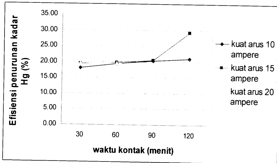
Gambar 4.3 Grafik hubungan Efisiensi penurunan kadar Hg dan waktu kontak pada kuat arus
