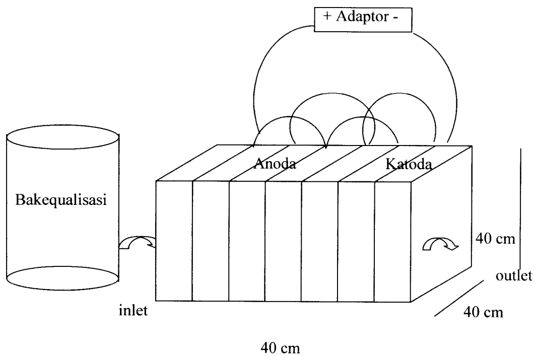
Gambar 3.4 Reaktor Elektrolisis
