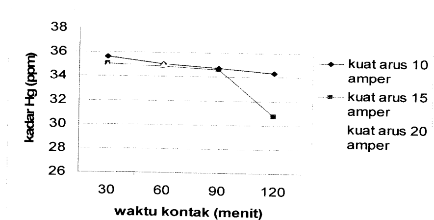
Gambar 4.1 Grafik hubungan kadar Hg dengan variasi waktu kontak pada kuat arus
