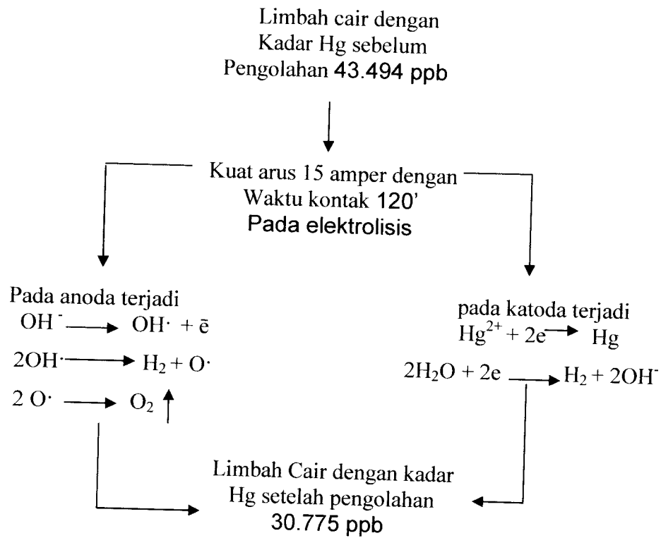
Gambar 4.5 Bagan fenomena yang terjadi pada proses elektrolisis
