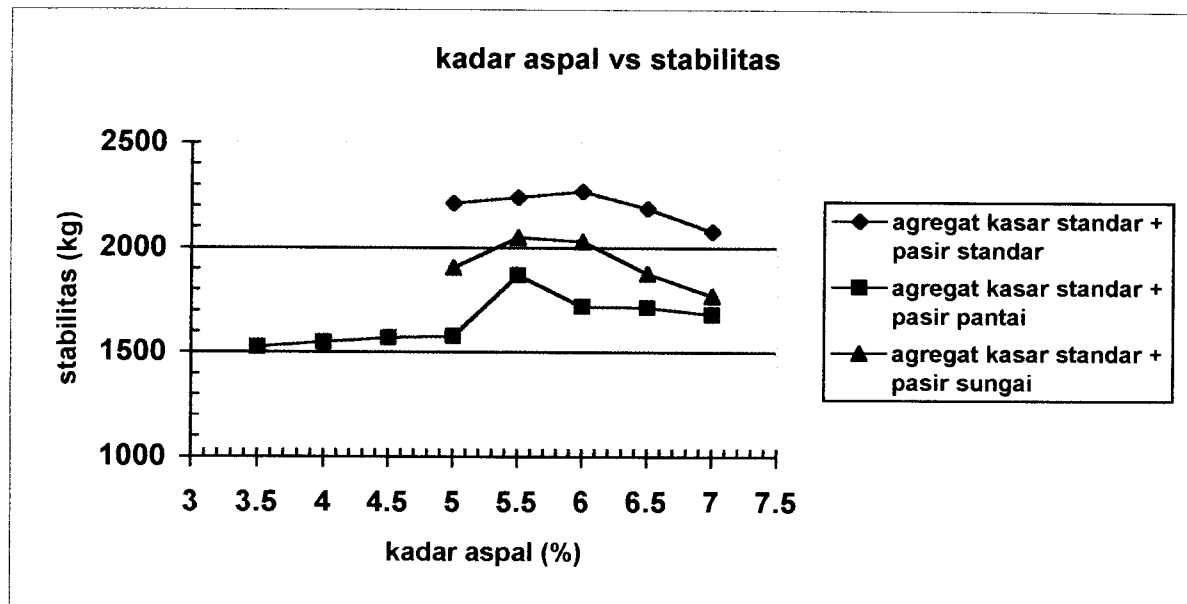
Gambar 6.5 Grafik hubungan antara kadar aspal dengan stabilitas
