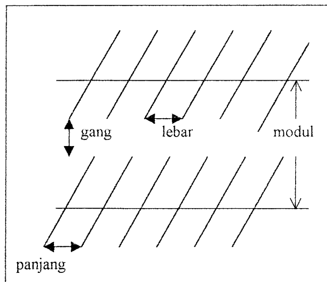
Gambar 3.14 Gang dan modul sudut parkir 30^\circ , 45^\circ dan 60^\circ
