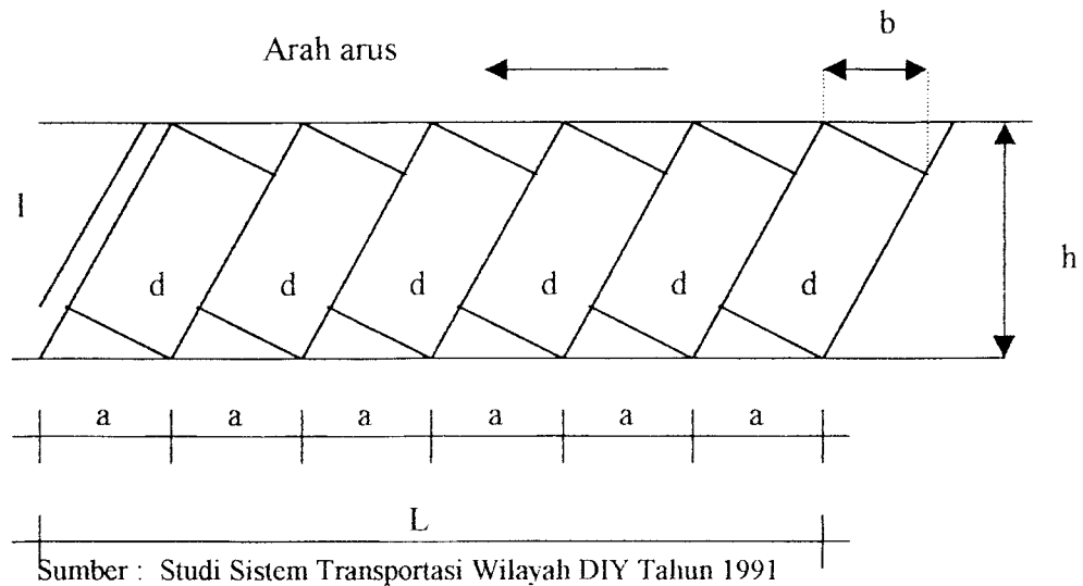
Gambar 3.9 Sketsa Ruang Parkir
