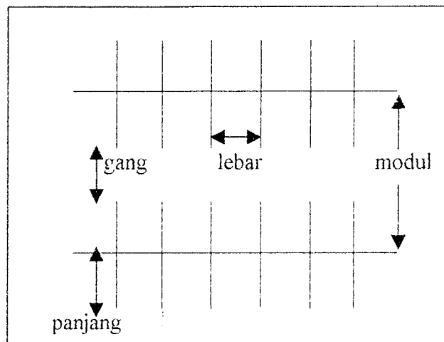
Gambar 3.13 Gang dan modul sudut parkir 90^\circ
