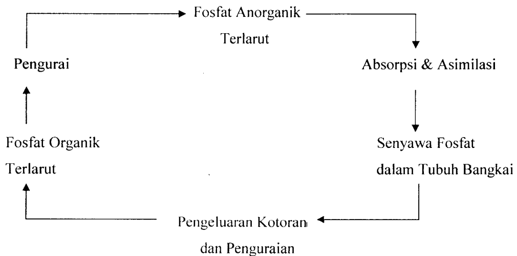
Gambar 2.2 Daur Fosfat
