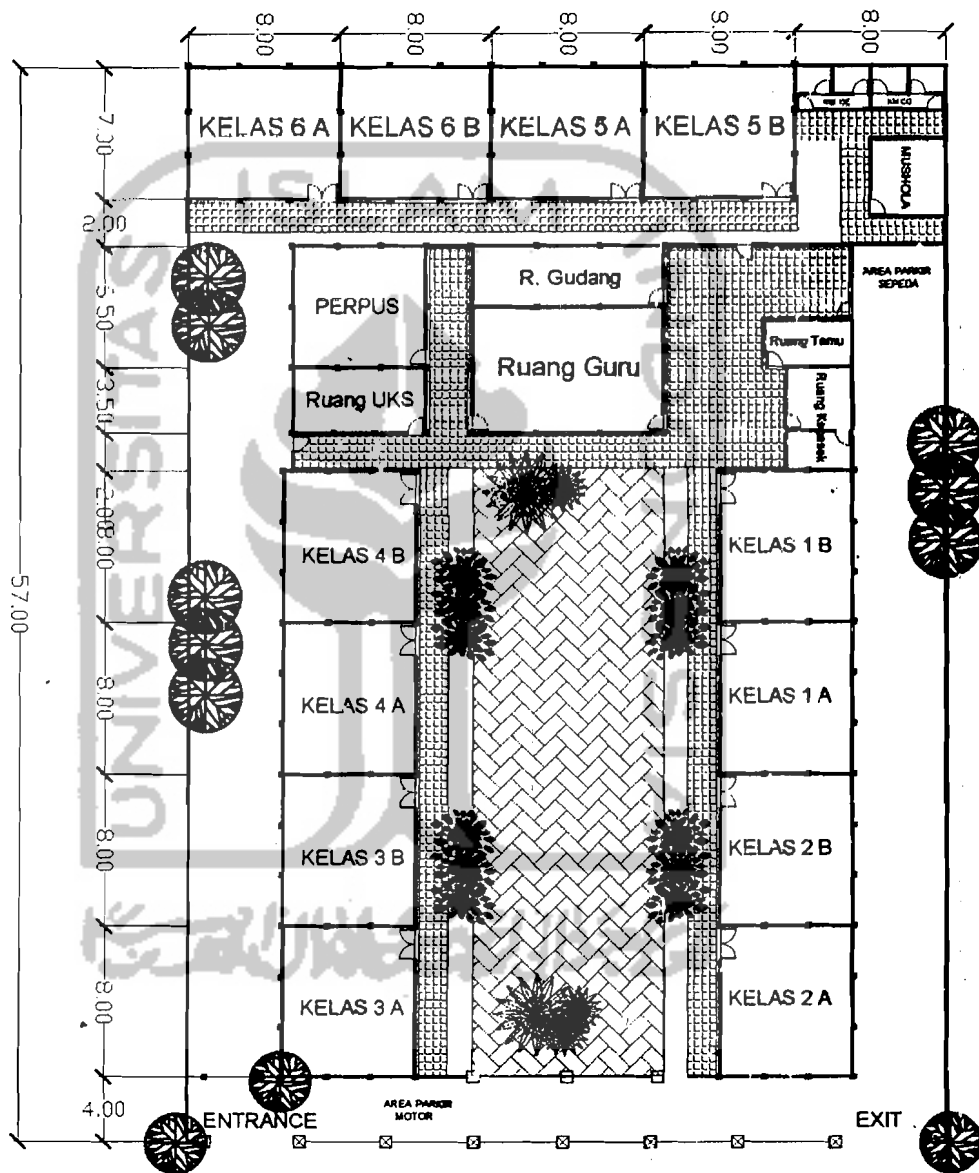
DENAH SDN 1 ADISUTJIPTO
