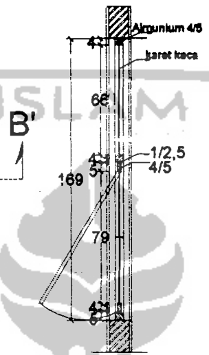
POTONGAN A-A' JENDELA HIDUP
