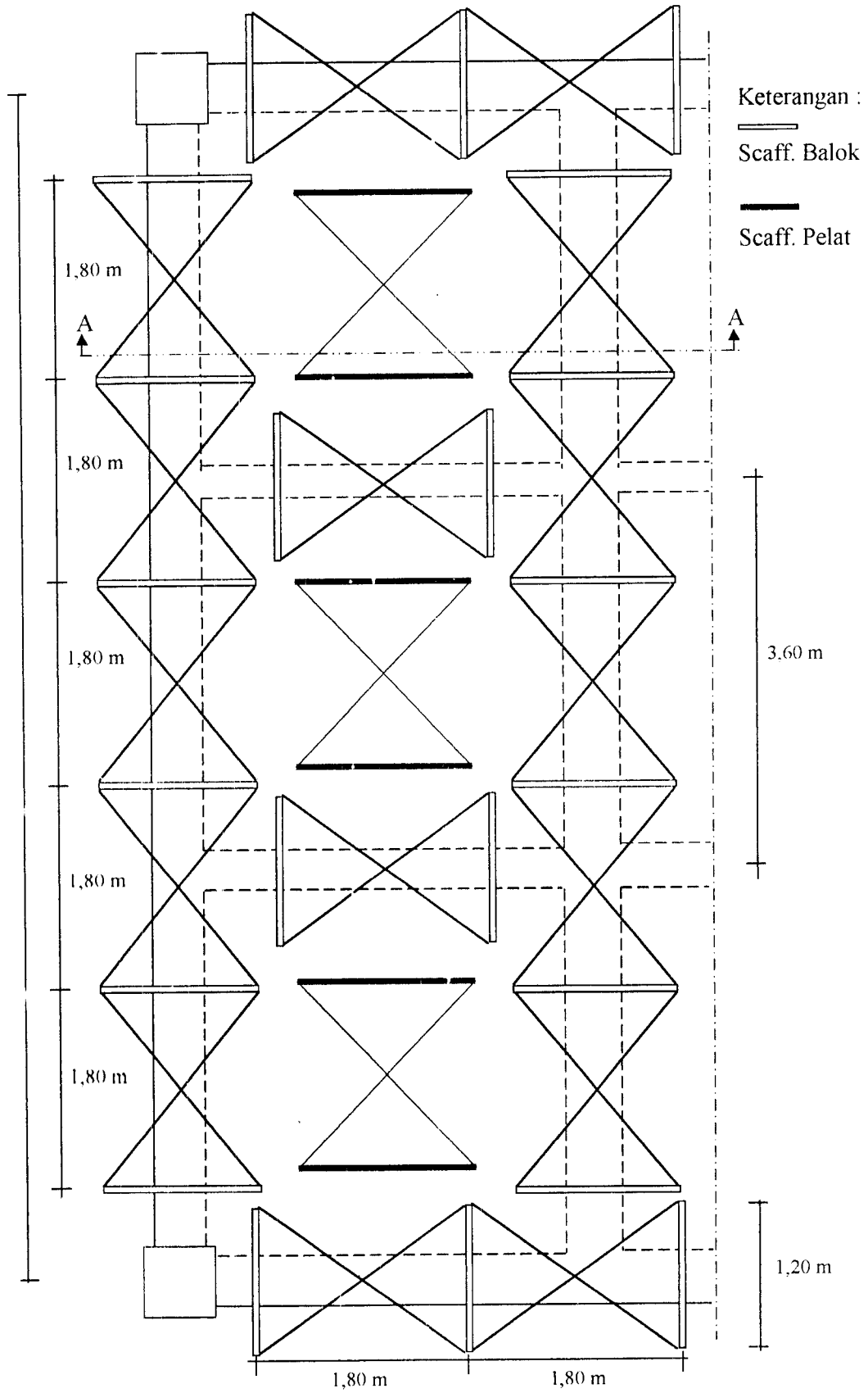
DENAH PENEMPATAN SCAFFOLDING BALOK DAN PELAT
