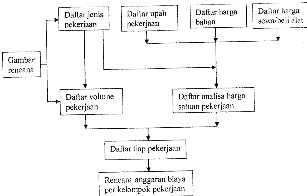
Gambar 3.3 Skema Perhitungan RAB dengan Metoda B.O.W Sumber : John W. Niron. Rencana Anggaran Biaya Bangunan, Jakarta, 1992.
