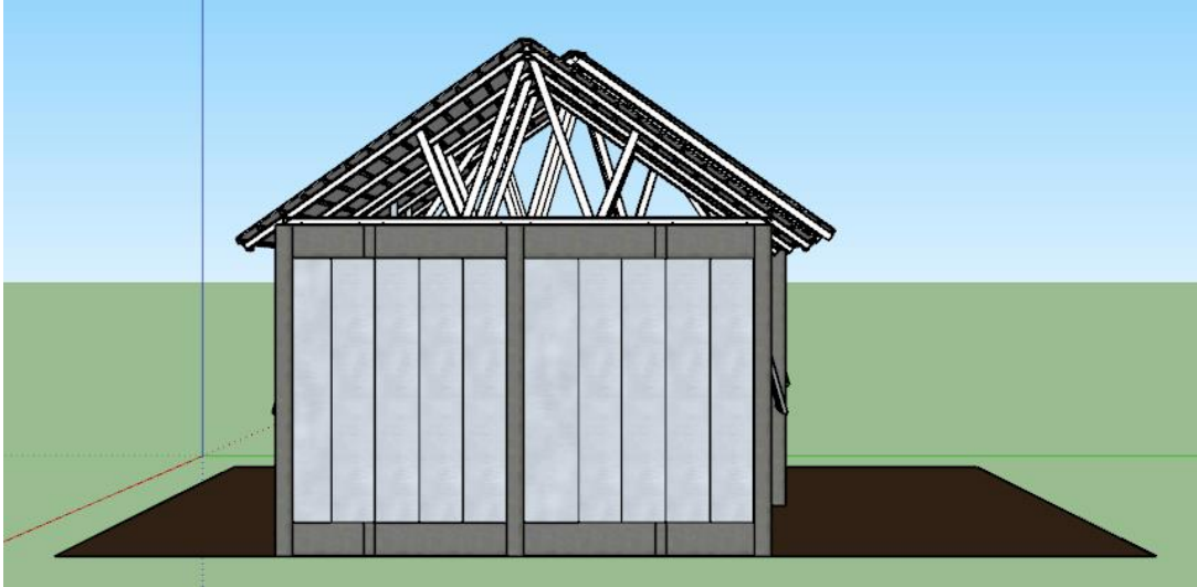
Tampilan Desain Usulan Rumah Subsidi Prefabrikasi (Sisi Kana)
