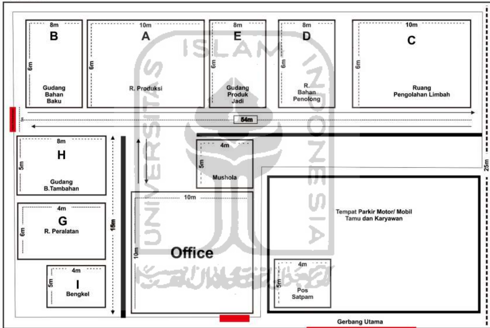
Layout Usulan :
