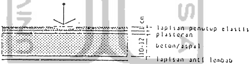
Gb. KONSTRUKSI ELASTIS TIDAK FLEKSIBLE
