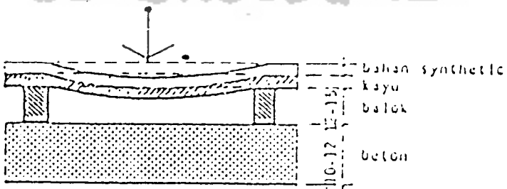
Gb. KONSTRUKSI ELASTIS FLEKSIBLE
