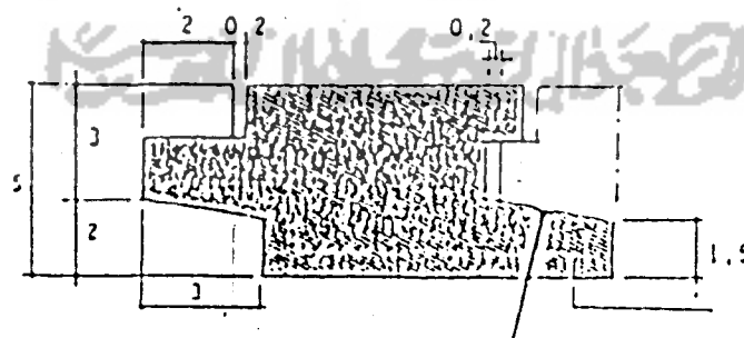
Gb. CONTOH DETAIL SAMBUNGAN LANTAI.
