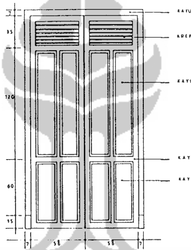
DETAIL PINTU D SKALA 1:20
