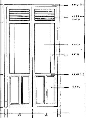
DETAIL PINTU E SKALA 1:20
