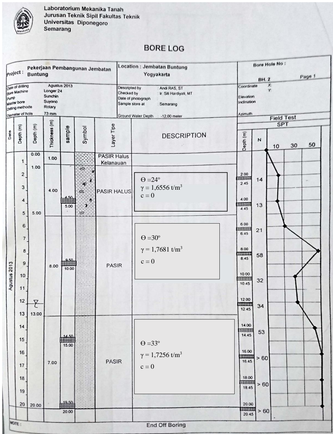
Gambar L-2.3 Data Tanah pada Kedalaman Pondasi
