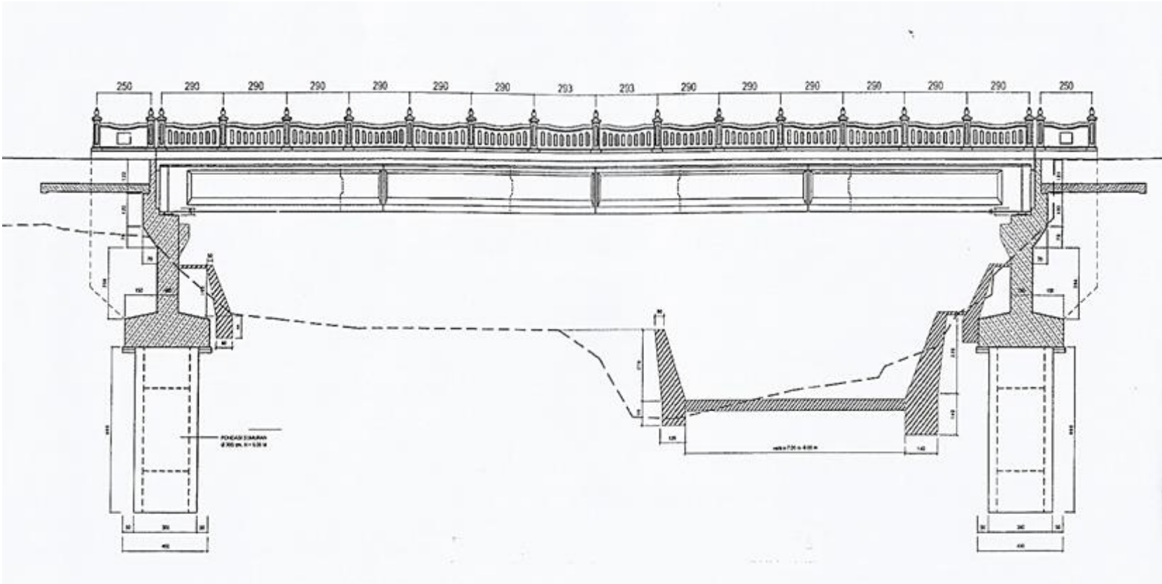
Gambar L-2.1 Potongan Memanjang Jembatan
