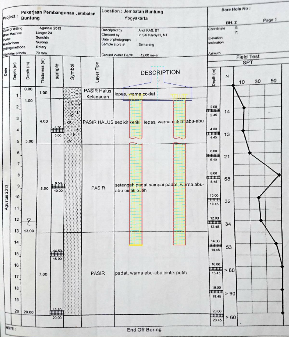
Gambar L-2.2 Teknis Perletakan Kedalaman Pondasi
