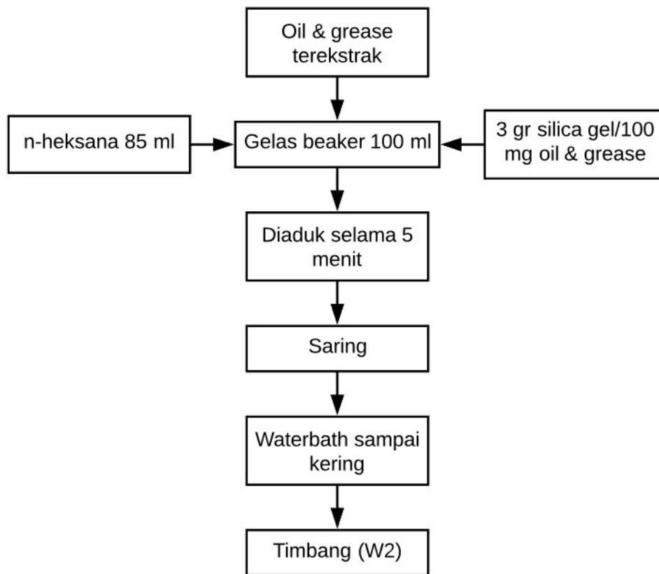
Diagram Alir Pengujian TPH
