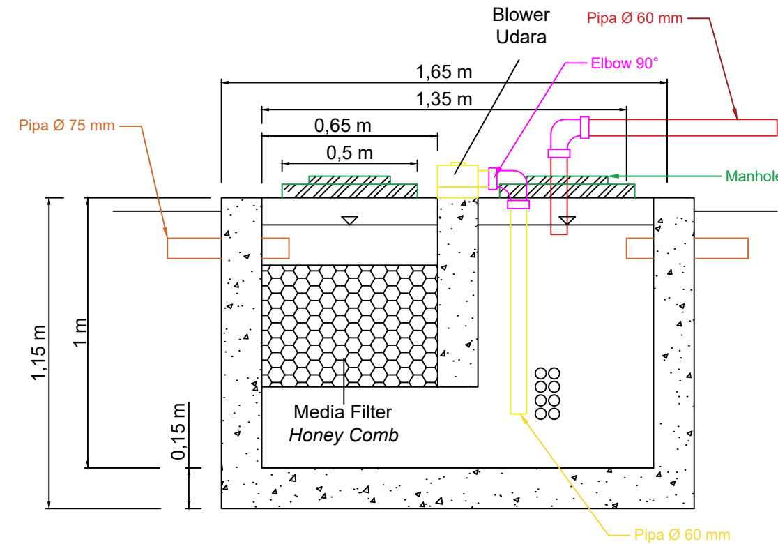
Potongan B - B Potongan Samping
