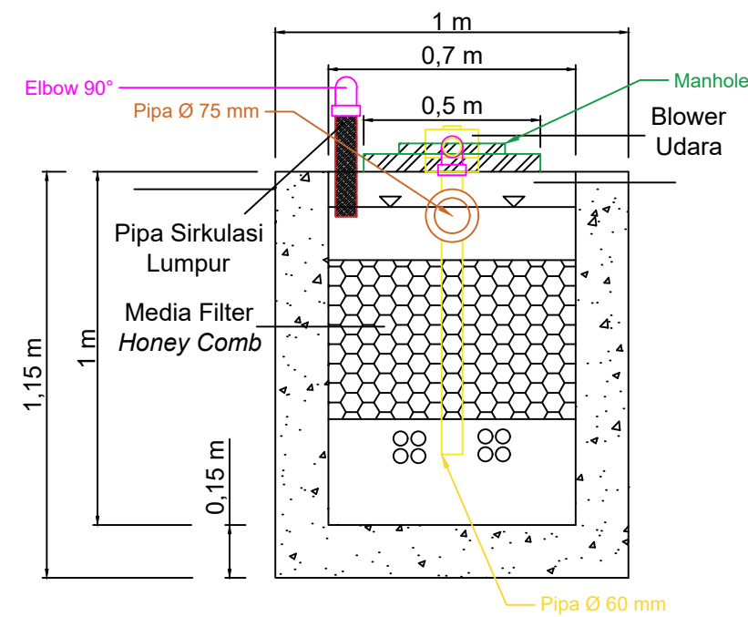
Potongan A - A Potongan Depan
