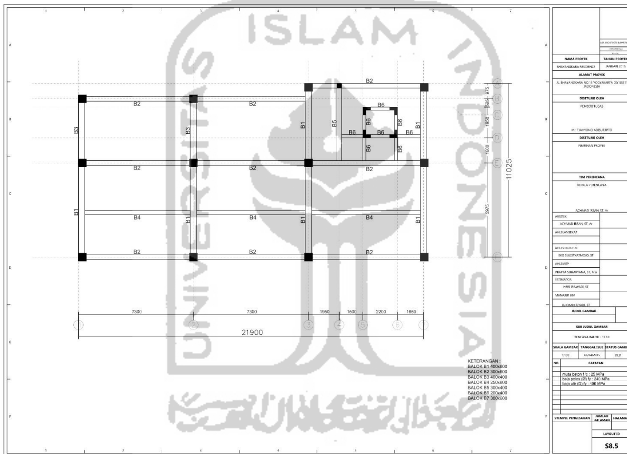
Gambar L-4.5 Denah Balok Lantai 6
