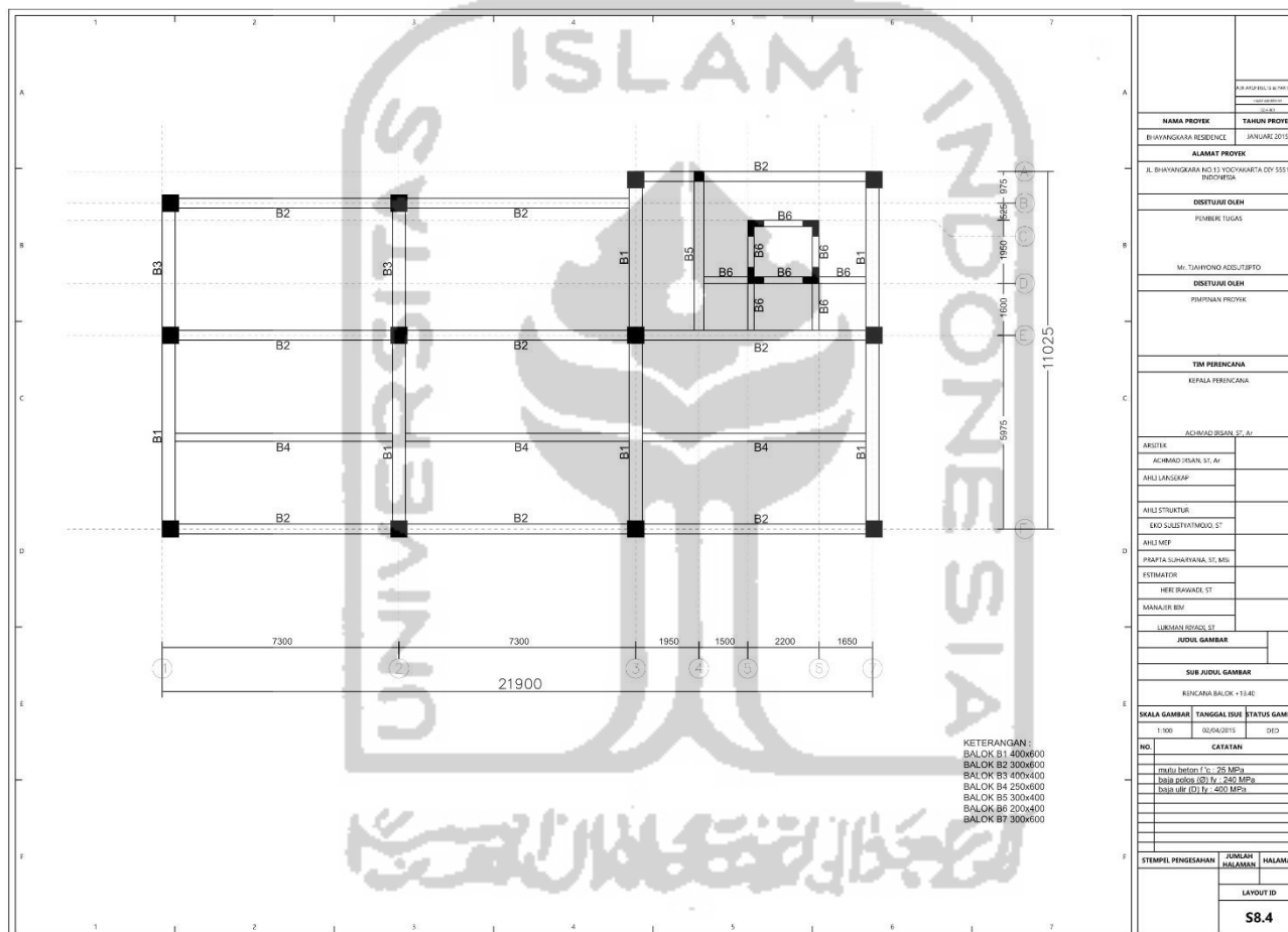
Gambar L-4.4 Denah Balok Lantai 5
