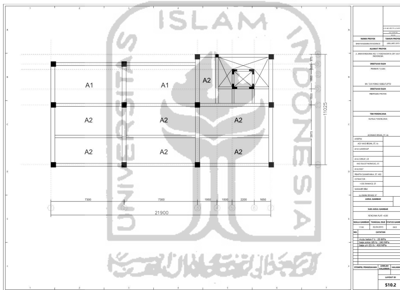
Gambar L-3.2 Denah Pelat Lantai 3
