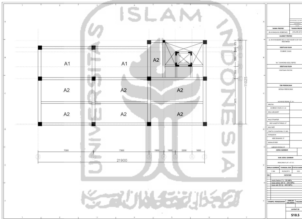
Gambar L-3.5 Denah Pelat Lantai 6
