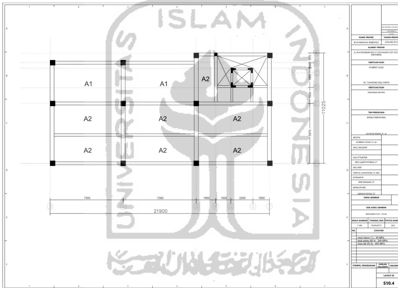
Gambar L-3.4 Denah Pelat Lantai 5
