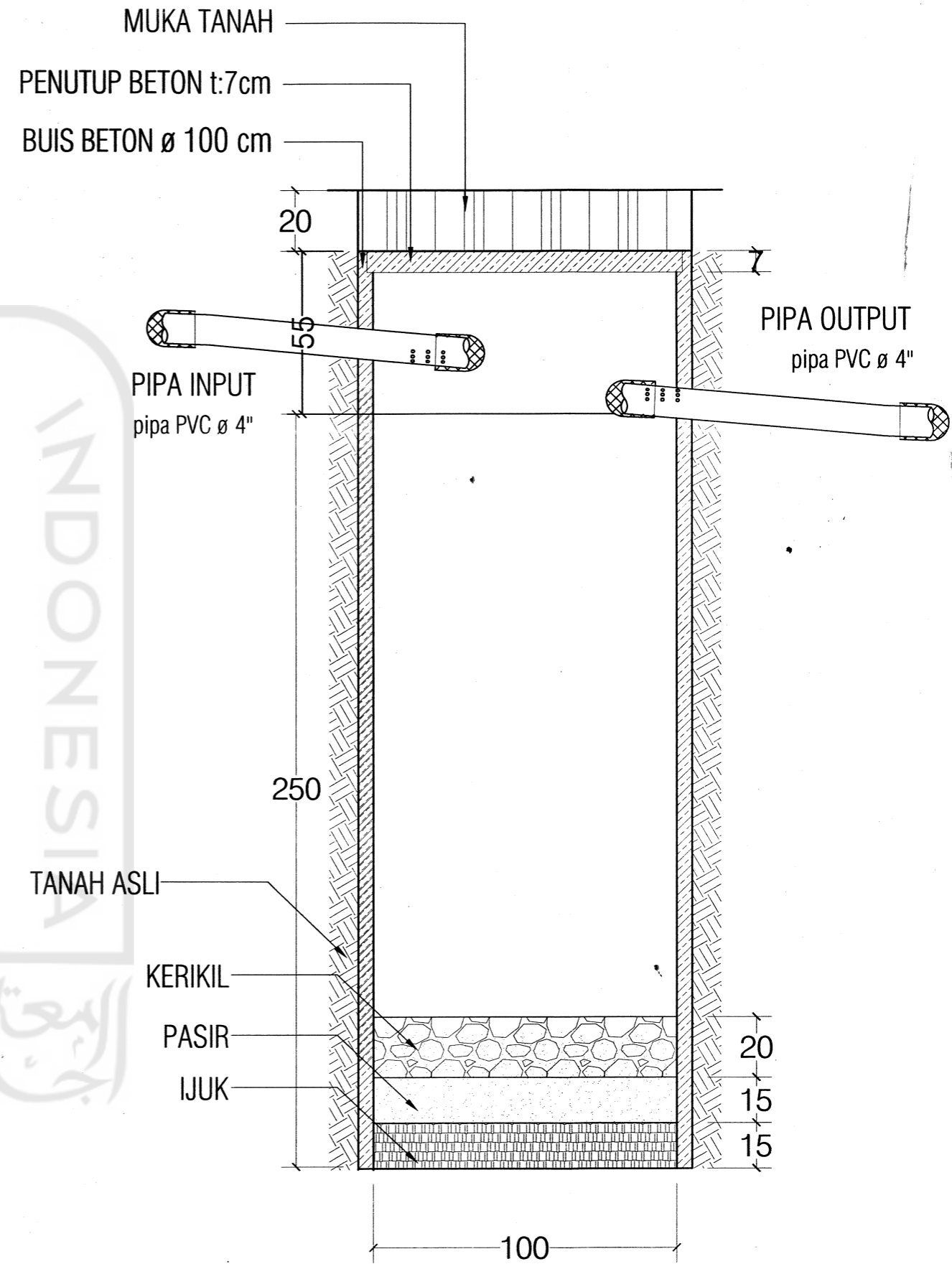
4 A-100 1 : 25 POTONGAN A - A
