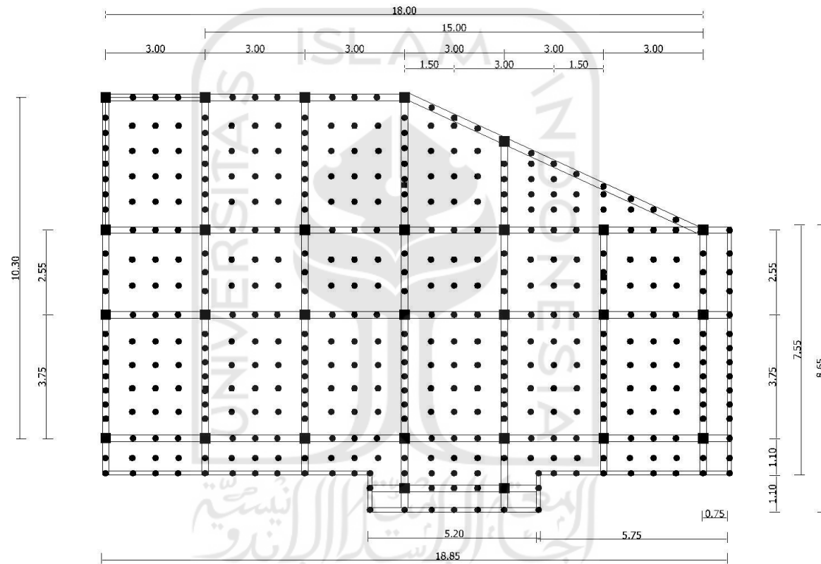
DENAH KEBUTUHAN BAMBU LANTAI 1 SKALA 1:100
