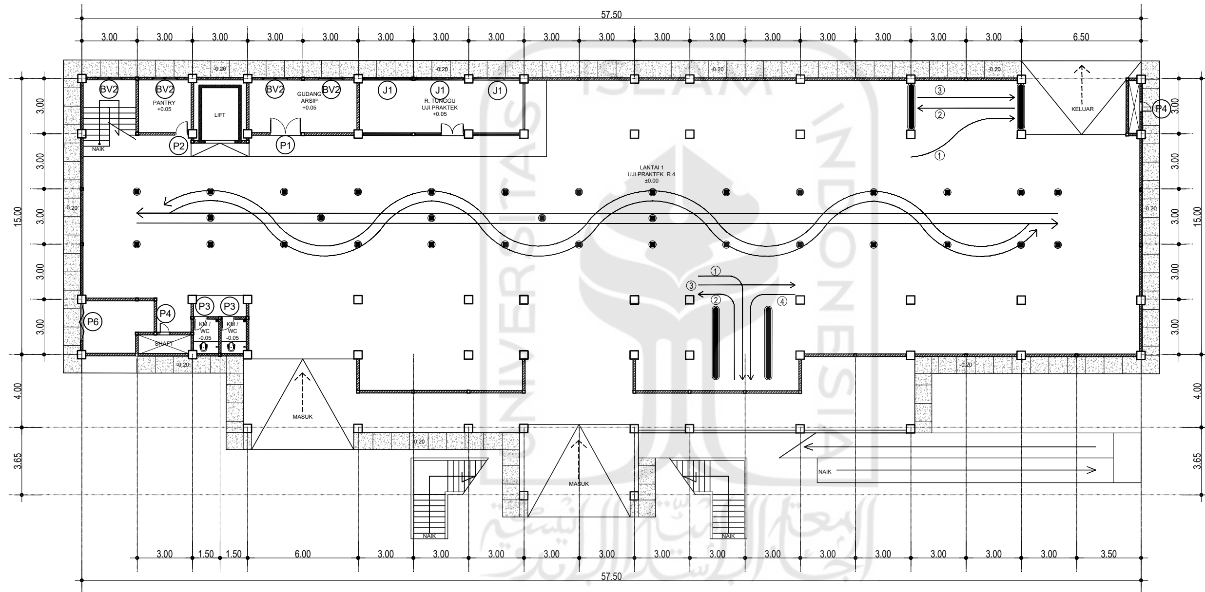
RENCANA PINTU JENDELA LANTAI 1 SKALA 1 : 200
