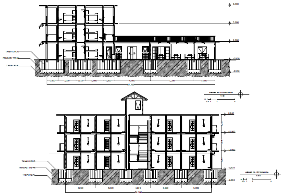
Gambar 4.14 Rancangan Sistem Struktur Potongan, Rencana Kolom Balok Asrama Santriwati dengan Pondasi Footplate. Sumber: Penulis (2019)
