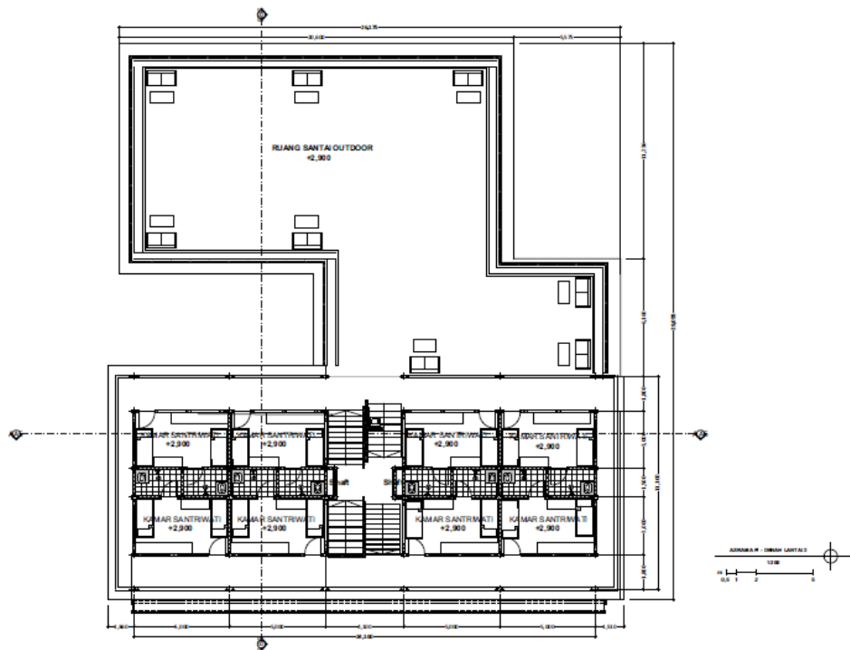
Gambar 4.2 Denah Asrama Santriwati Lantai 1 dan Lantai 2 (Atas ke bawah) Sumber: Penulis (2019)
