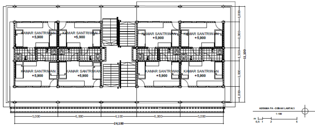
Gambar 4.3 Denah Asrama Santriwan Lantai 1, Lantai 2 dan Lantai 3 (Atas ke bawah) Sumber: Penulis (2019)
