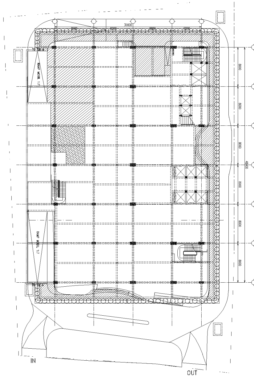
Gambar L-3.1 Denah Struktur Lantai Dasar
