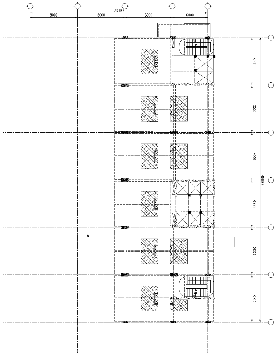
Gambar L-3.2 Denah Struktur Lantai 7-20
