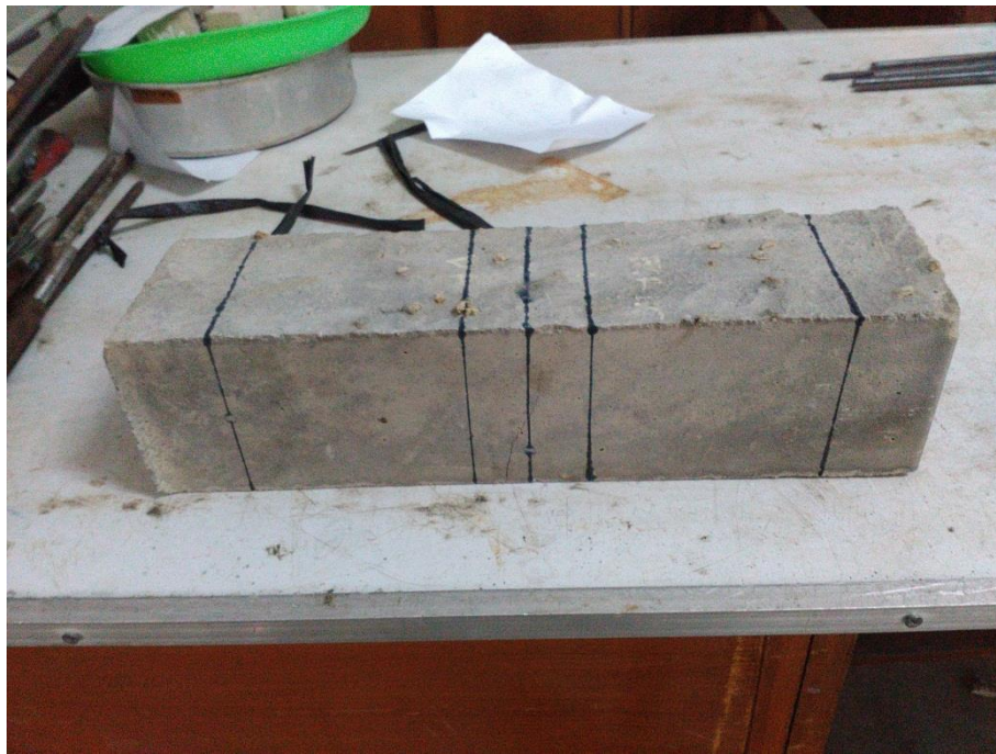
Gambar L-8.5 Pola Retakan Balok Beton BSR 2
