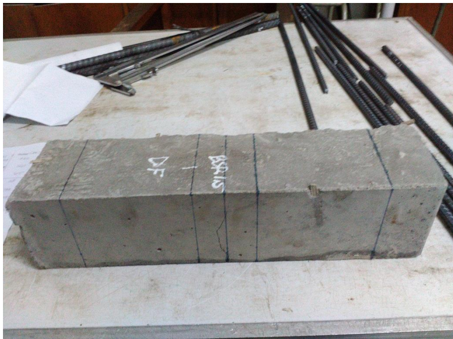
Gambar L-8.4 Pola Retakan Balok Beton BSR 1,5
