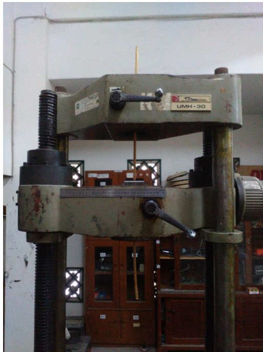
Gambar L-3.4 Pengujian Kuat Tarik Rotan
