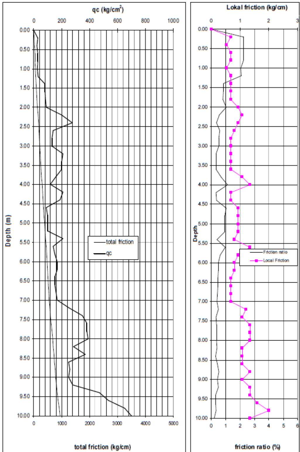
Gambar 3.2 Grafik Hasil Uji Sondir Titik 2
