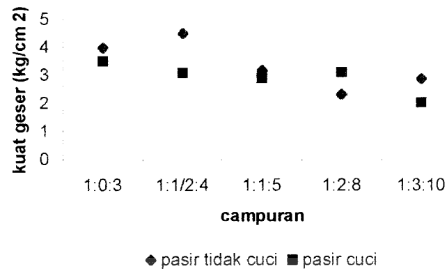
Gambar 5.7 Grafik Kuat Geser Pasangan Bata
