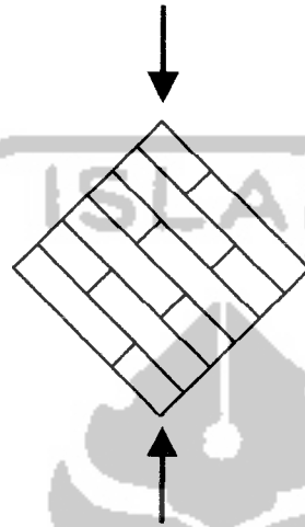
Gambar 3.7 Gambar Benda Uji Geser Pasangan Bata
