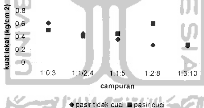
Gambar 5.6 Grafik Kuat Lekatan Mortar dan Bata
