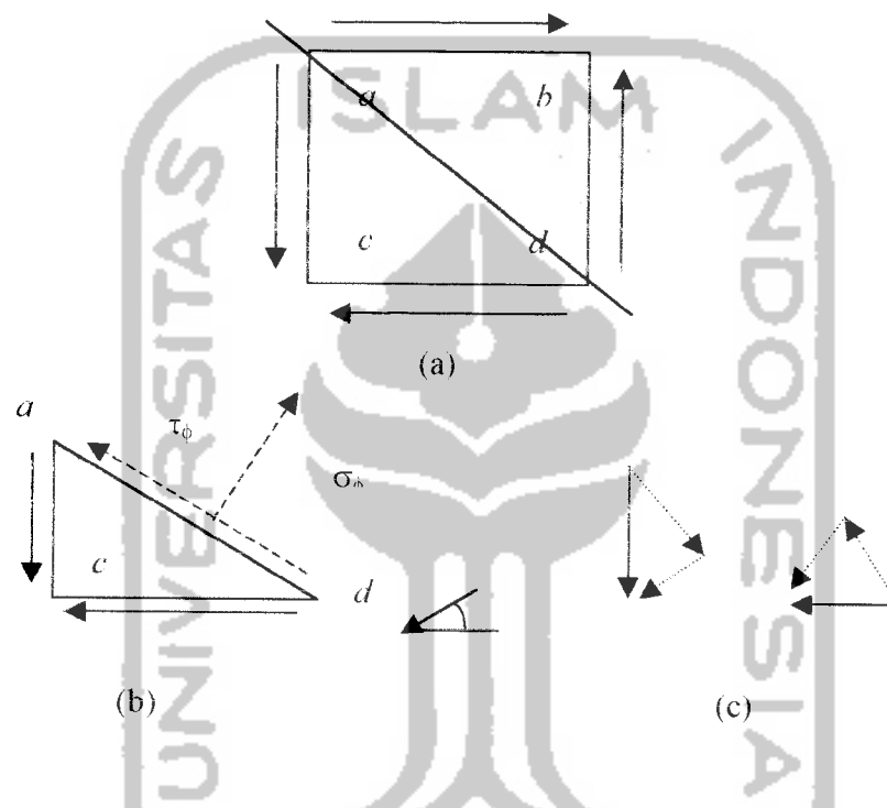
Gambar 3.2 Analisa Tegangan pada Bidang Miring
