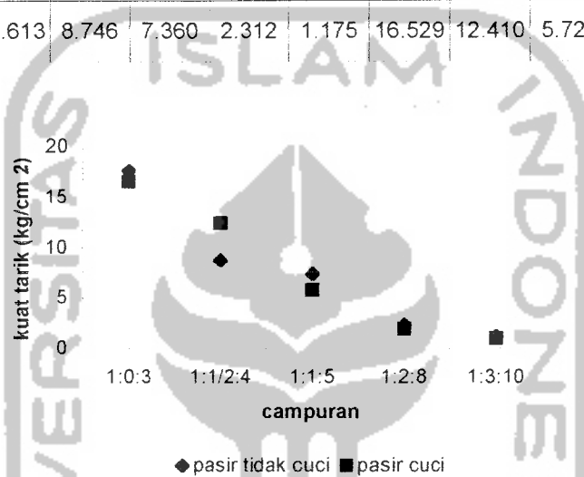
Gambar 5.5 Grafik kuat Tarik Mortar
