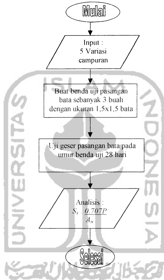
Gambar L.11 Bagan Alir Geser Pasangan
