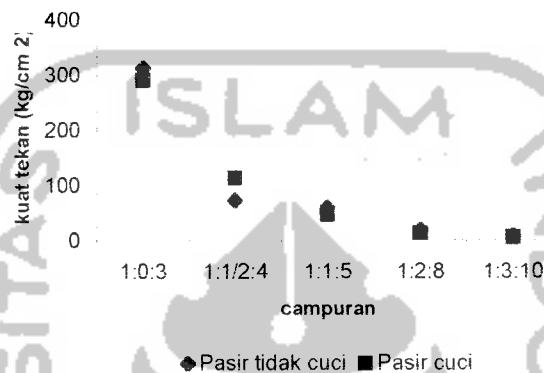
Gambar 5.4 Grafik Kuat Tekan Mortar
