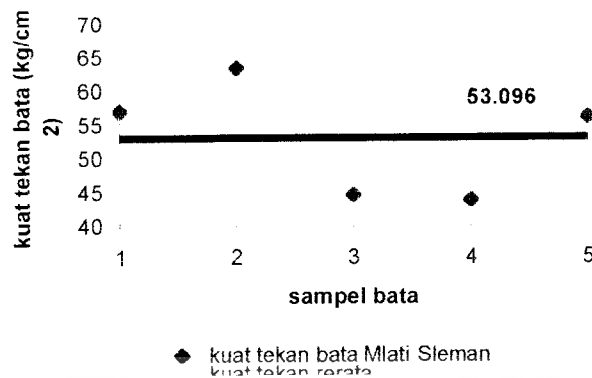
Gambar 5.2 Grafik Kuat Tekan Bata
