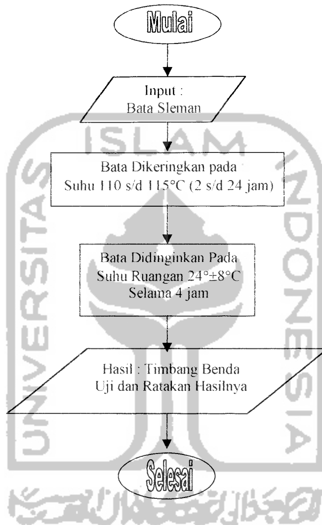
Gambar L.2 Bagan Alir Berat Bata
