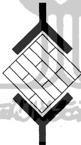
Gambar 3.14 Gambar Pengujian Kuat Geser Pasangan Bata
