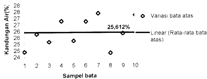
Gambar 5.3 Grafik Uji Serapan Air
