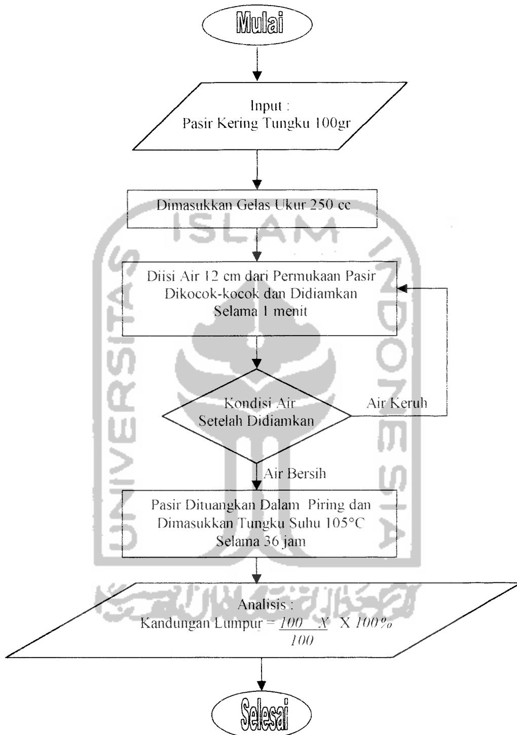
Gambar L.7 Bagan Alir Pemeriksaan Kandungan Lumpur Dalam Pasir
