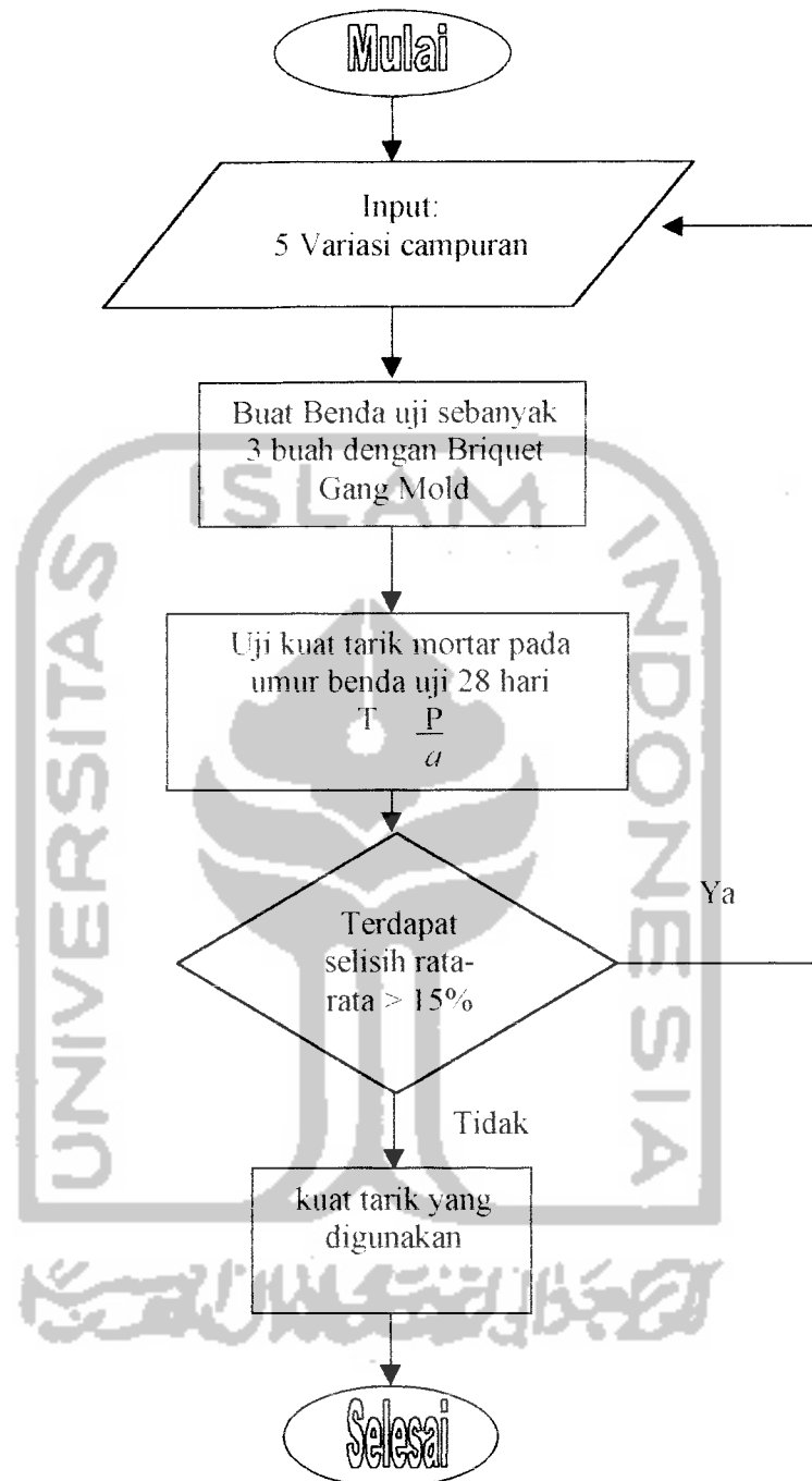
Gambar L.9 Bagan Alir Tarik mortar
