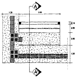
DENAH HALTE 1:50
