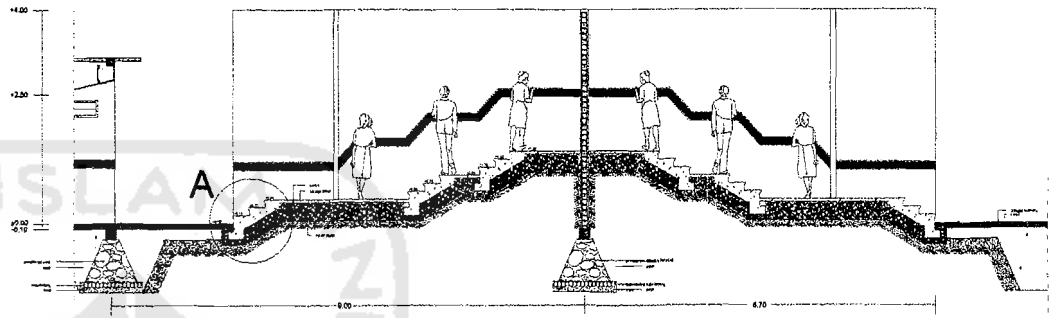
POTONGAN A-A' 1:50
