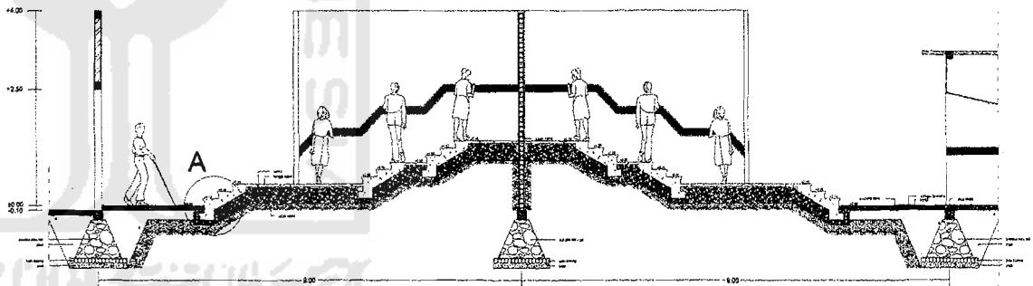
POTONGAN B-B' 1:50
