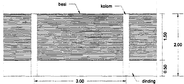
TAMPAK PAGAR 1 1:25
