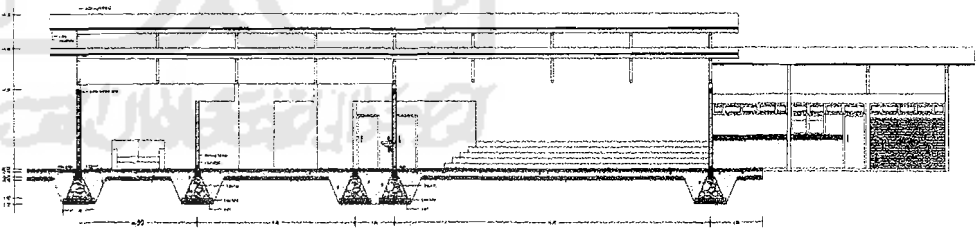
POTONGAN B-B'
