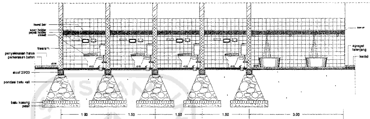
POTONGAN A-A' 1:25
