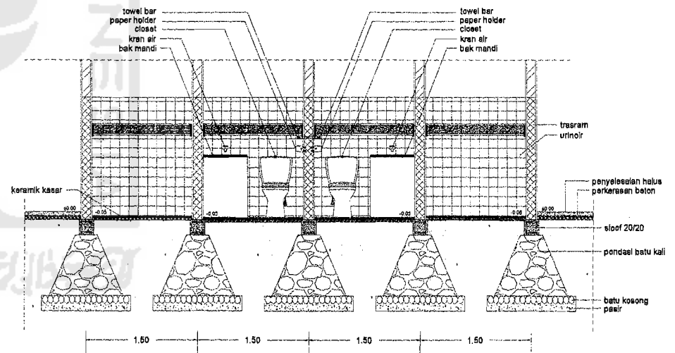
POTONGAN C-C' 1:25
