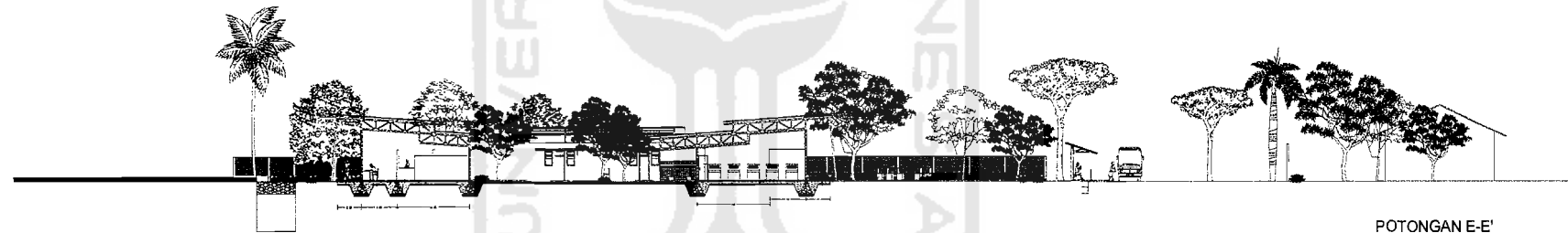
POTONGAN E-E'
