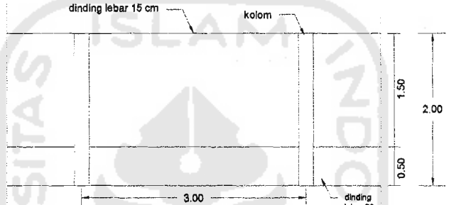
TAMPAK PAGAR 2 1:25
