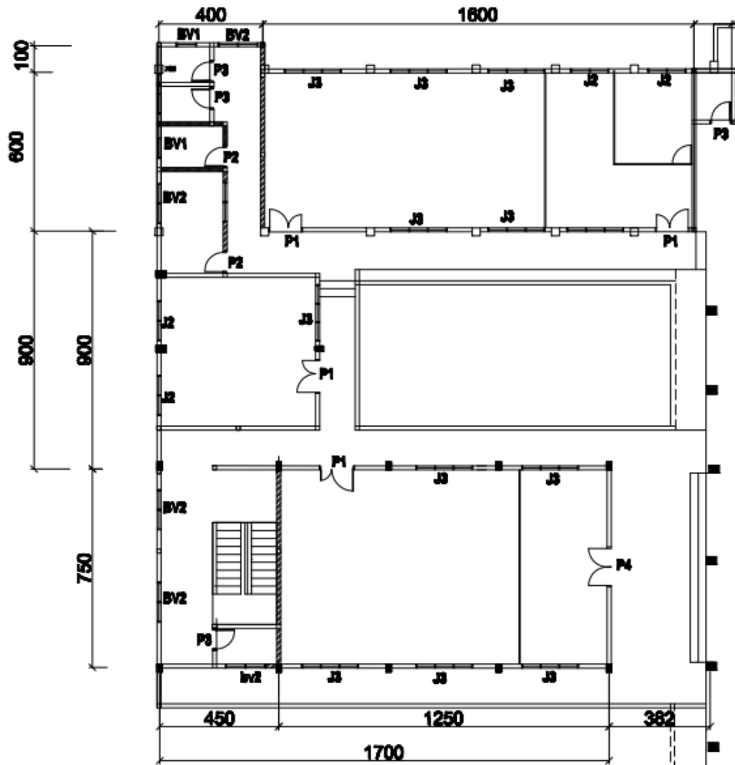
Lanjutan Lampiran 1. Gambar Denah Lantai 2
