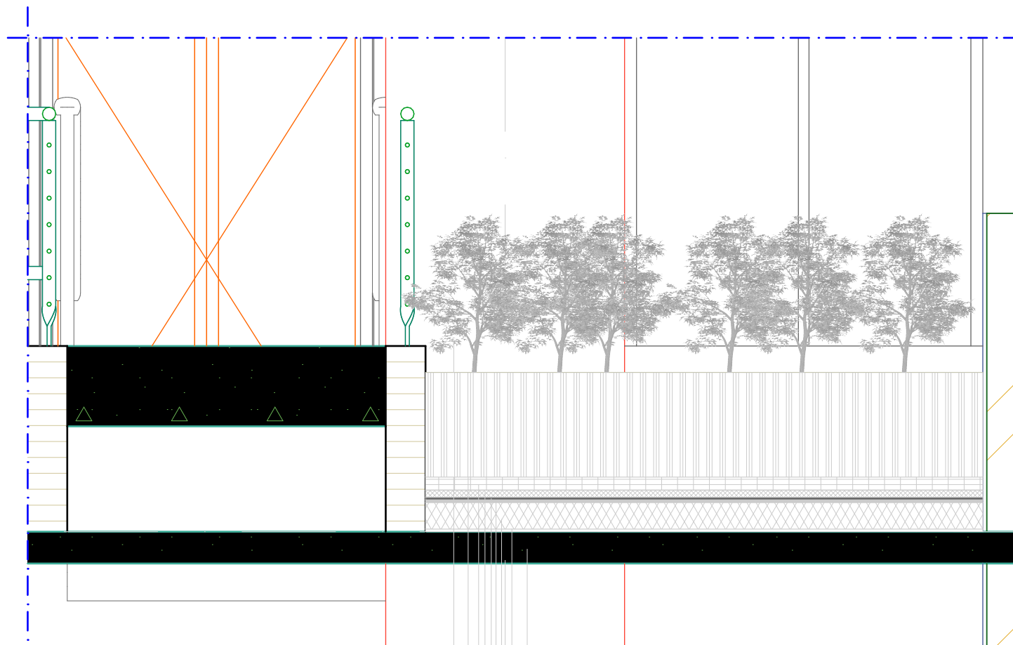
DETAIL KONSTRUKSI ROOF FARMING
