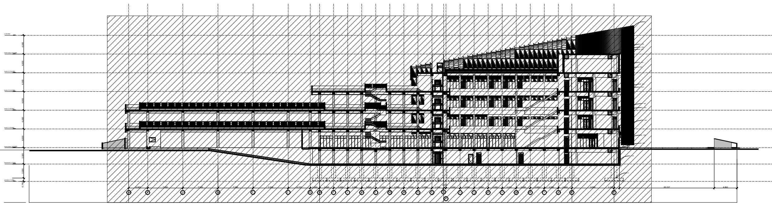
POTONGAN E-E 1 : 500
