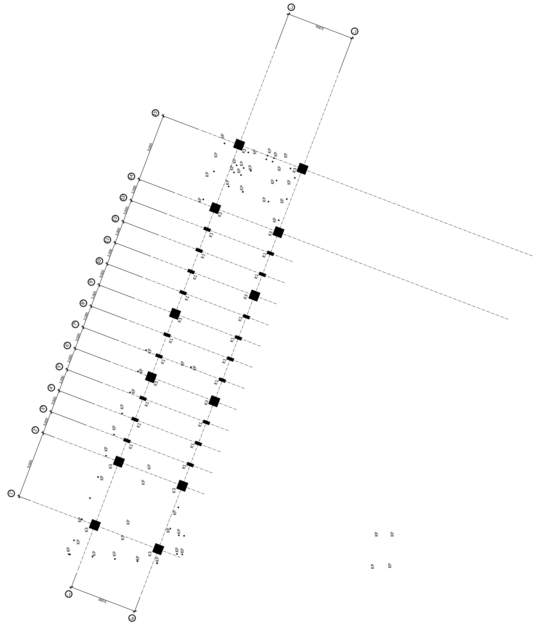
RENCANA KOLOM lantai 4 1 : 300
