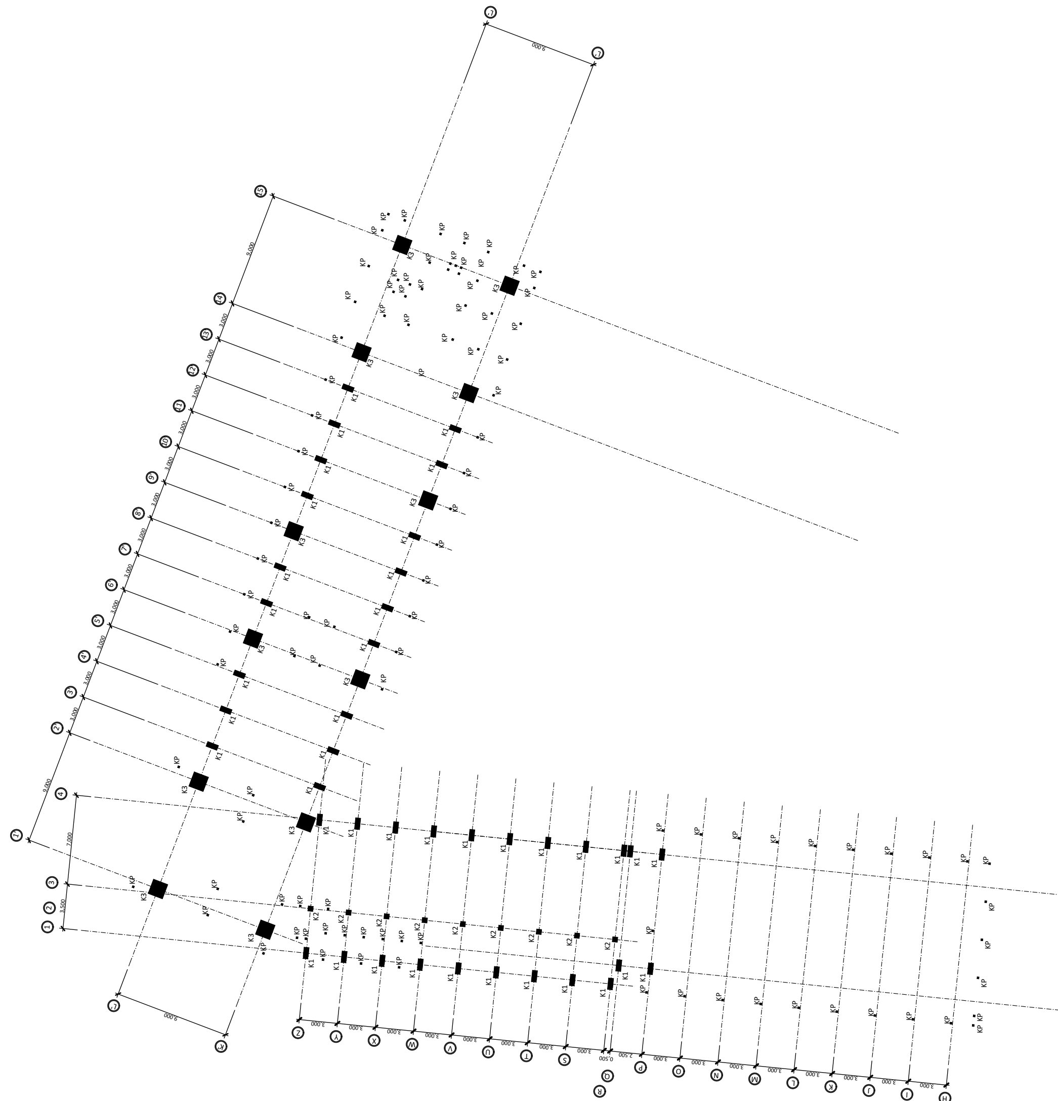
RENCANA KOLOM lantai 3 1 : 300
