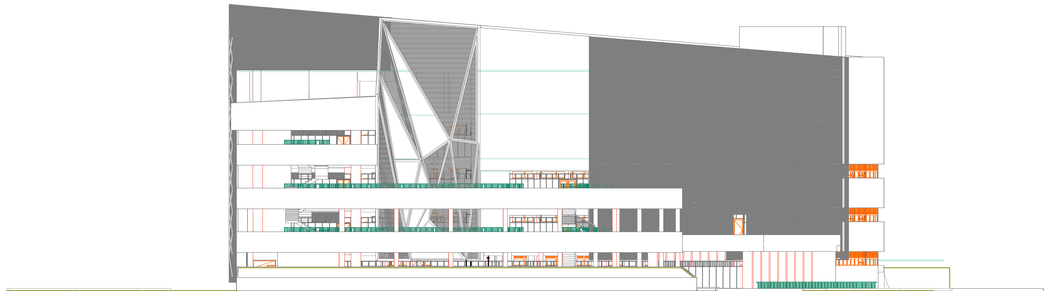
TAMPAK SELATAN 1 : 200
