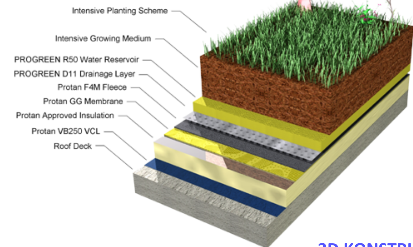
3D KONSTRUKSI ROOF FARMING
