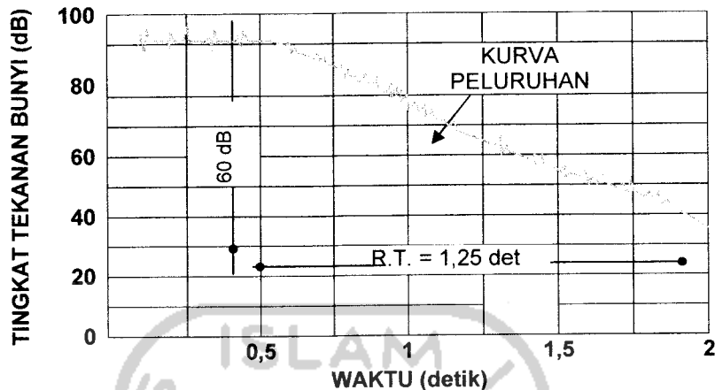
Gambar 2.2 Waktu dengung (RT) suatu ruang didefinisikan sebagai waktu yang dibutuhkan suatu bunyi yang tiba-tiba dihentikan untuk berkurang dengan 60 dB. (sumber : Akustik Lingkungan )
