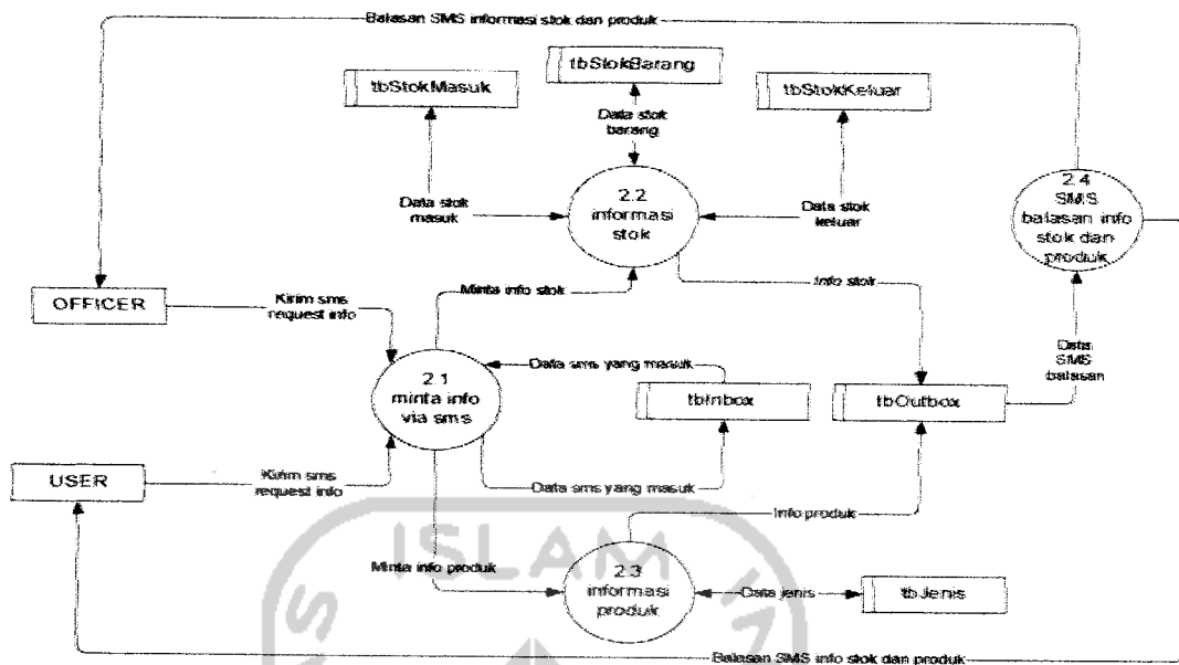
Gambar 4.4 DFD Level-2 Proses-2 Info Stok dan Produk via SMS
