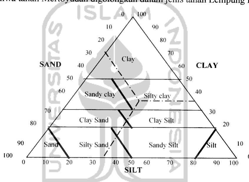
Gambar 5.3 Klasifikasi Tanah Mertoyudan Menurut USCS
