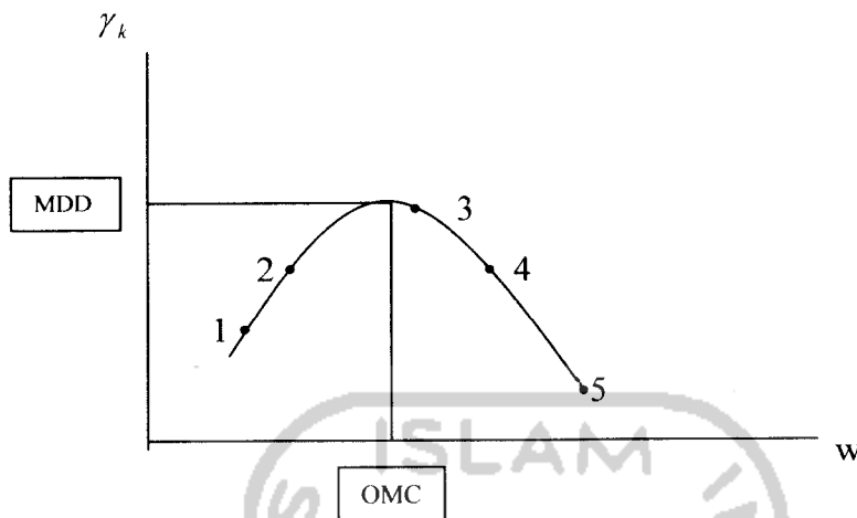
Gambar 4.3 Grafik hubungan \gamma_k dengan kadar air ( w )
