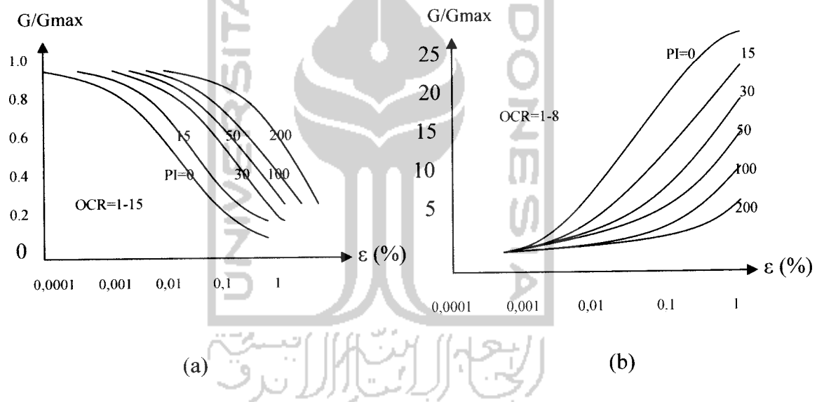
Gambar 2.1 Hubungan antara G/G_{max} lawan regangan geser (Sumber : Joseph E. Bowles (Analisis dan Desain Pondasi Jilid 1))
