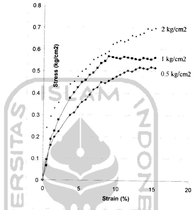
Gambar 6.1 Grafik Hubungan Tegangan dengan Regangan (Lampiran no. 21)
