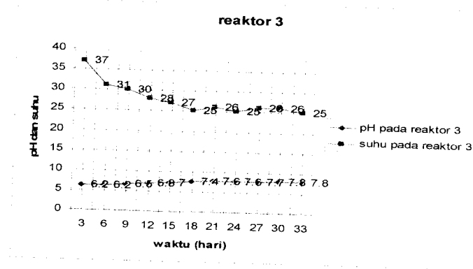
Gambar 4.13 Grafik Hubungan Suhu dan pH di Reaktor 3
