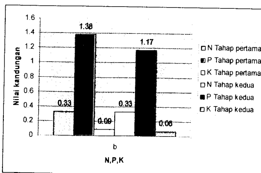
Gambar 4.20 Pengukuran N,P,K pada reaktor 2
