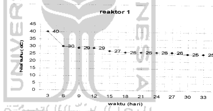
Gambar 4.7 Grafik Nilai Suhu di Reaktor 1
