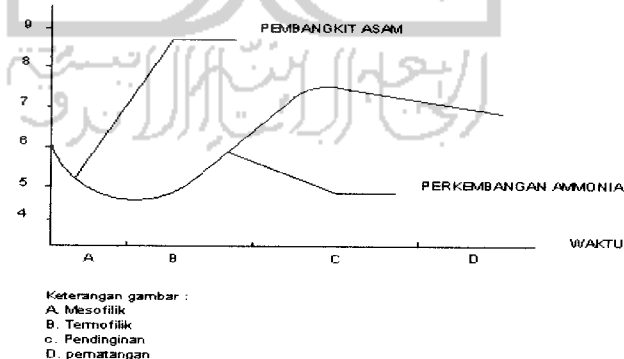
Gambar 2.2 Variasi pH dalam Tumpukan Kompos ( Dalzell, 1991 )
