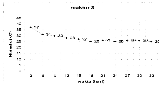
Gambar 4.9 Grafik Nilai Suhu di Reaktor 3
