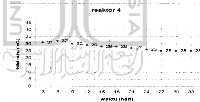
Gambar 4.10 Grafik Nilai Suhu di Reaktor 4
