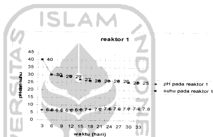
Gambar 4.11 Grafik Hubungan Suhu dan pH di Reaktor 1 Selama Proses Pengomposan
