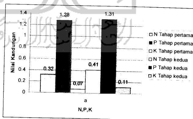
Gambar 4.19 Pengukuran N,P,K pada reaktor 1
