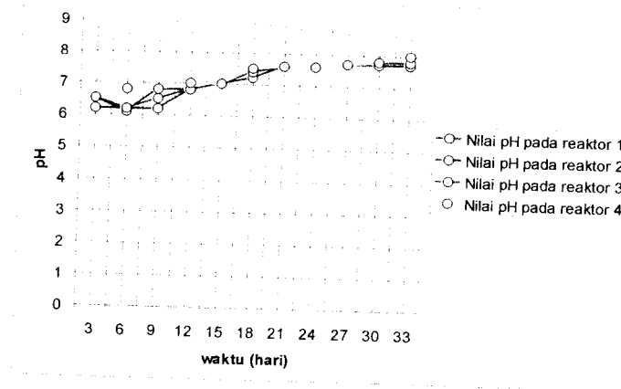
Gambar 4.1 Grafik Nilai pH Gabungan Selama Proses Pengomposan
