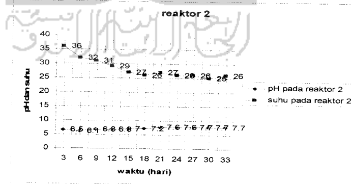
Gambar 4.12 Grafik Hubungan Suhu dan pH di Reaktor 2 Selama Proses Pengomposan
