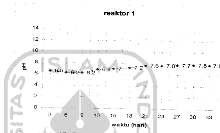
Gambar 4.2 Grafik Nilai pH di Reaktor 1 Selama Proses Pengomposan
