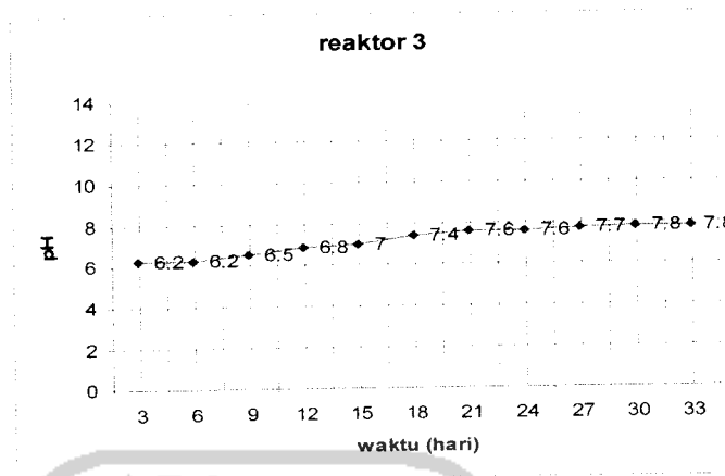
Gambar 4.4 Grafik Nilai pH di Reaktor 3
