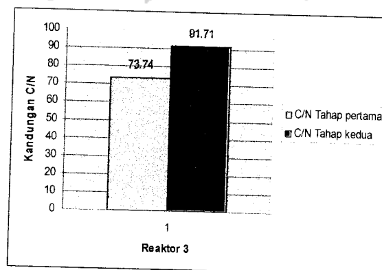
Gambar 4.17 Ratio C/N Pada Reaktor 3
