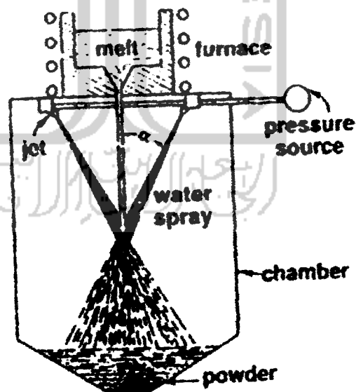
Gambar 2.8. Metoda atomisasi air [4].
