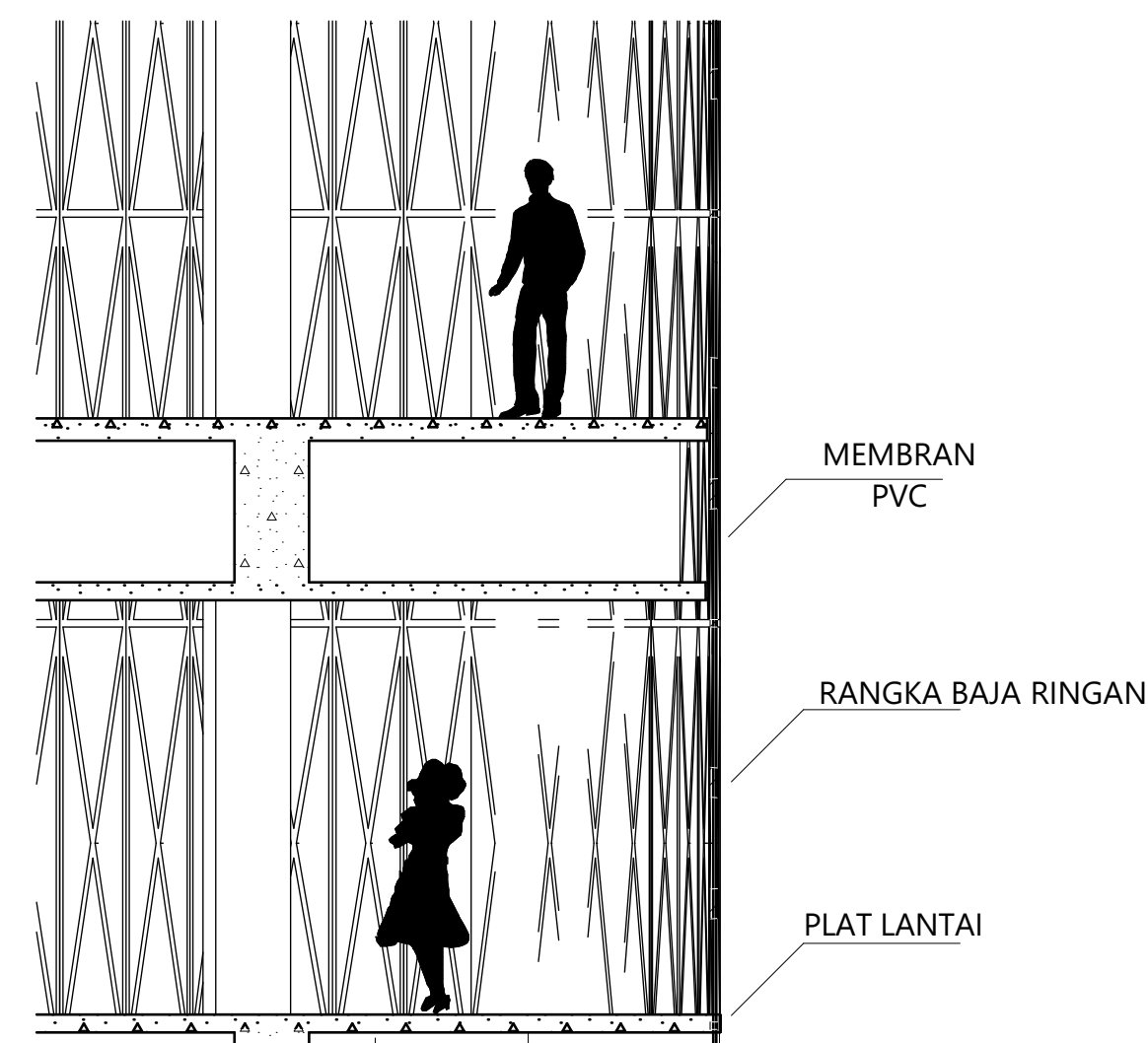
POTONGAN 10-10 1:100
