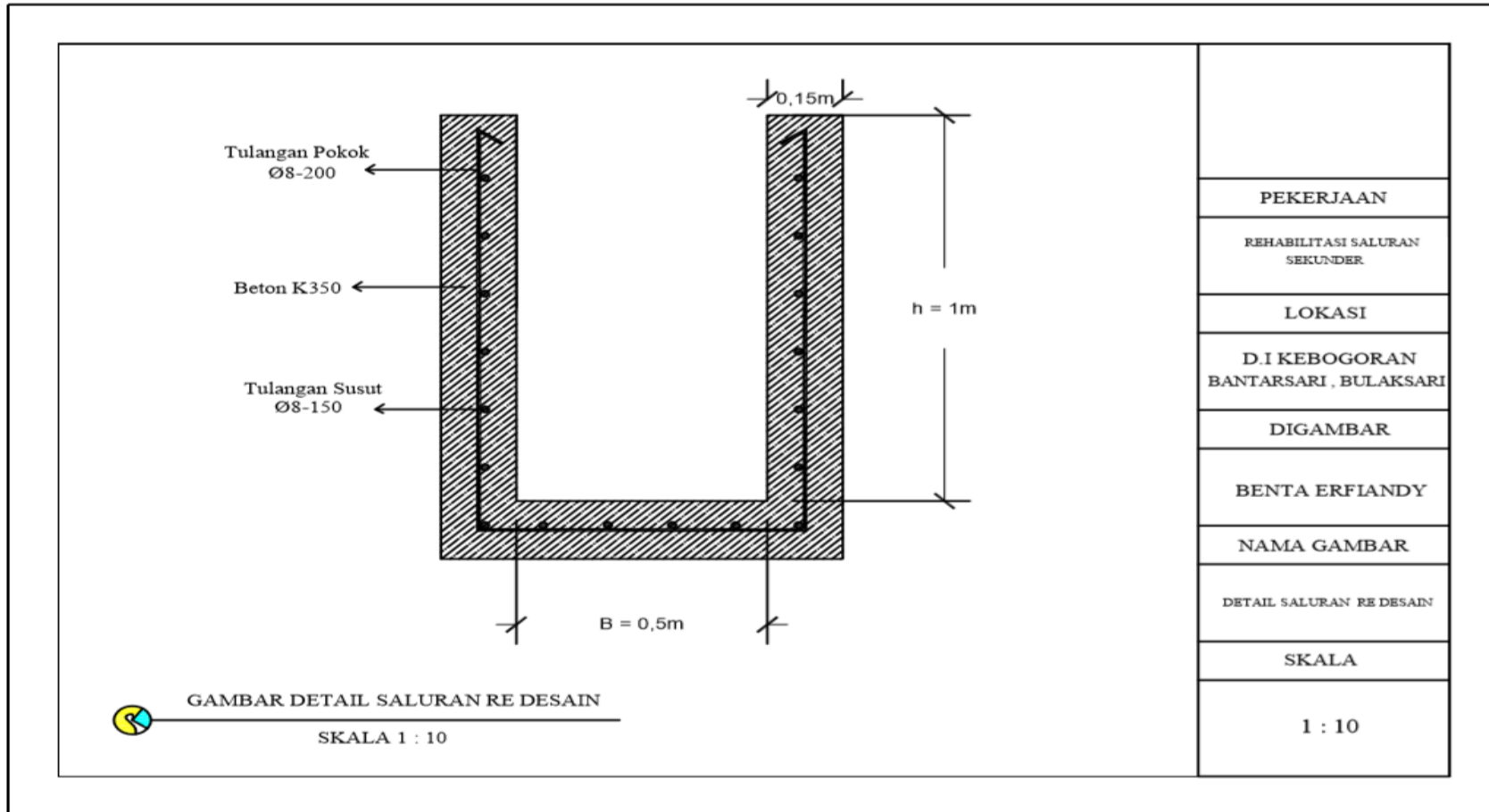
Lampiran 9. Gambar Detail Saluran Beton Bertulang Re- Desain
