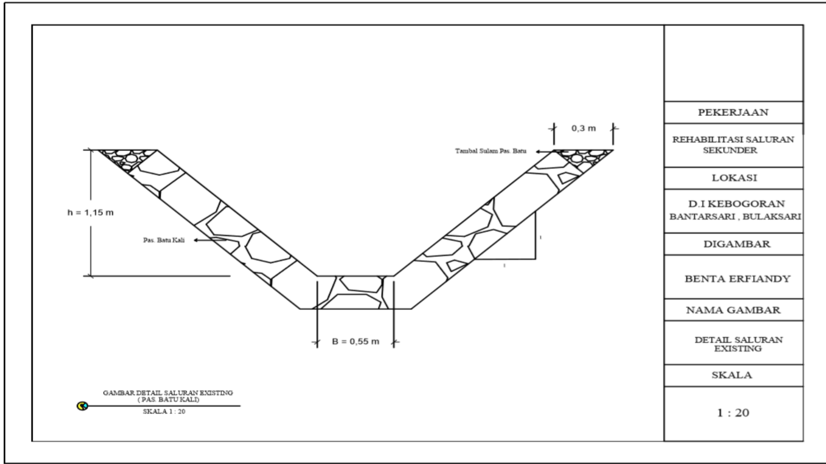
Lampiran 13. Gambar Detail Saluran Batu Kali ( Existing )
