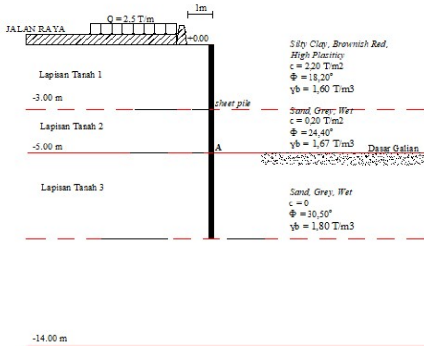
Gambar L-2.2 Pemodelan Potongan Melintang Galian
