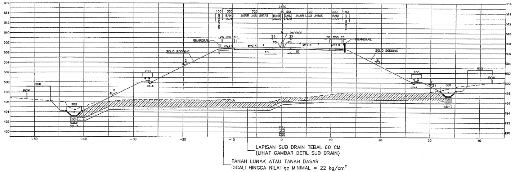
Gambar L-2 DED Timbunan Sta 46+000
