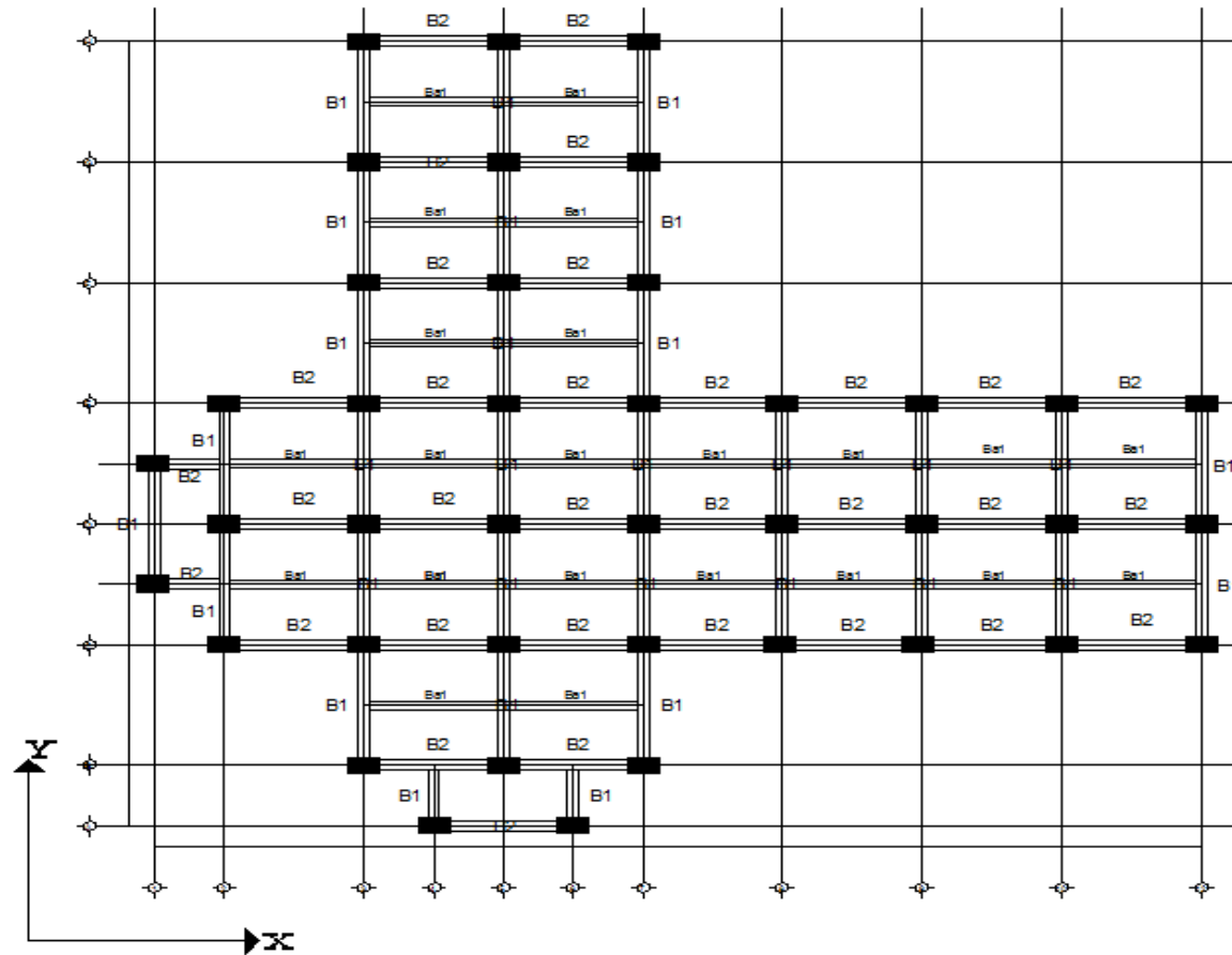
Gambar L-1.2 Denah Balok Model 2
