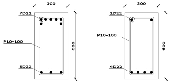
BALOK B2 DAERAH TUMPUAN (POT I-I) SKALA 1 : 10 BALOK B2 DAERAH LAPANGAN (POT II-II) SKALA 1 : 10
