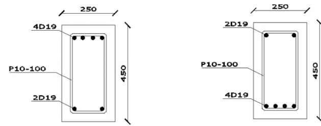
BALOK Ba1 DAERAH TUMPUAN (POT I-I) SKALA 1 : 10 BALOK Ba1 DAERAH LAPANGAN (POT II-II) SKALA 1 : 10
