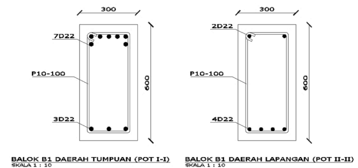
Gambar L-2.8 Penulangan Balok B1 Model 4 Lt. 7-9
