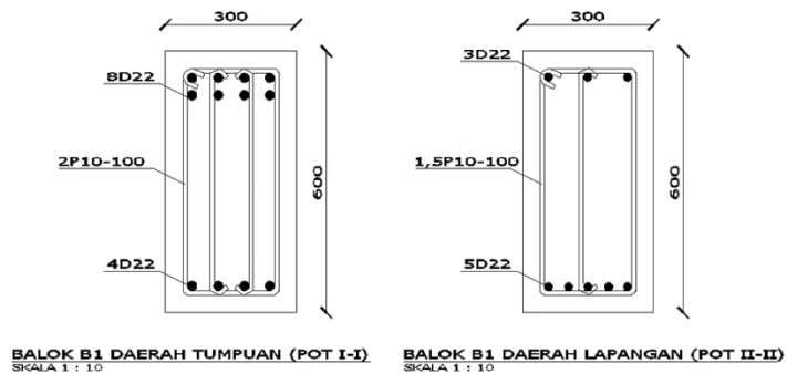
Gambar L-2.5 Penulangan Balok B1 Model 3 Lt. 1-6
