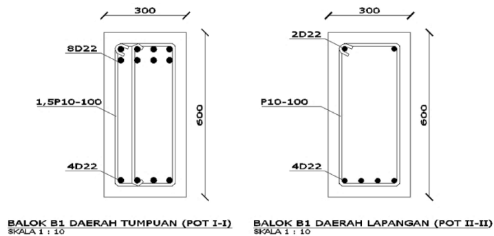
Gambar L-2.7 Penulangan Balok B1 Model 4 Lt. 1-6
