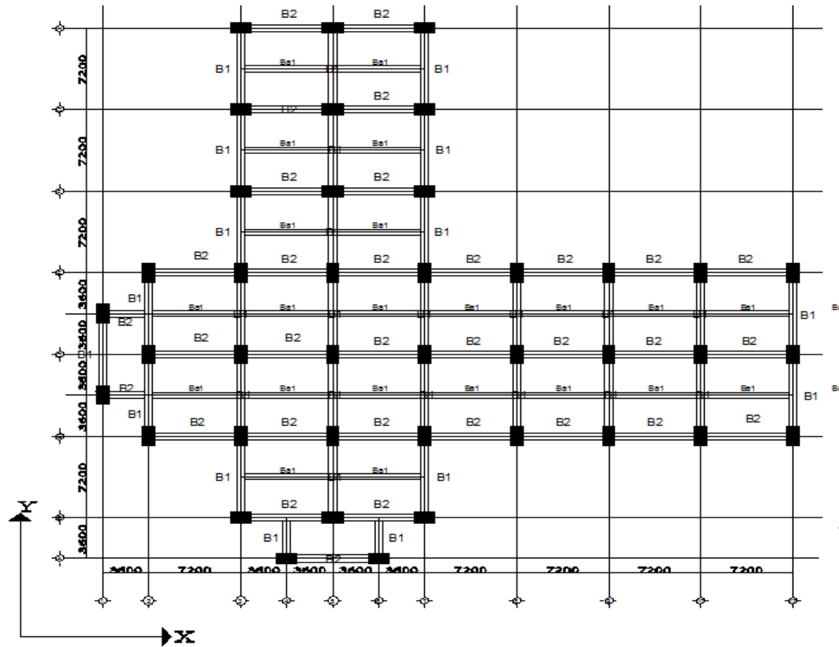
Gambar L-1.4 Denah Balok Model 4
