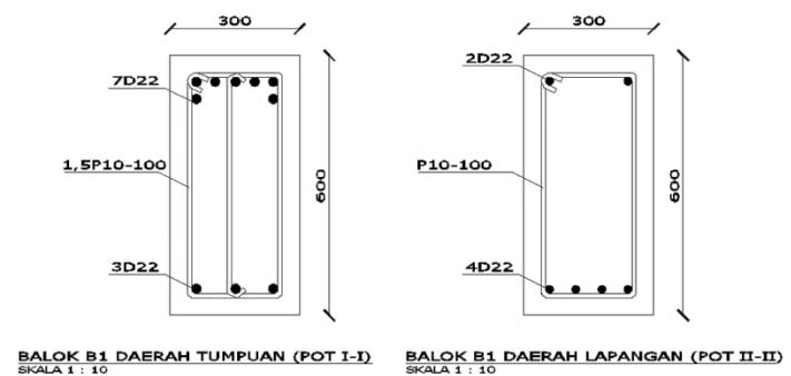
Gambar L-2.6 Penulangan Balok B1 Model 3 Lt. 7-9
