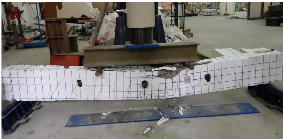
GAMBAR 16 BENDA UJI BALOK BERTULANG SETELAH DI UJI LENTUR
