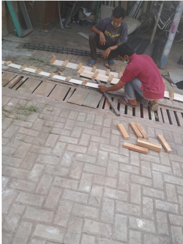
GAMBAR 11 PEMBUATAN BEKISTING BALOK DAN PENULANGAN
