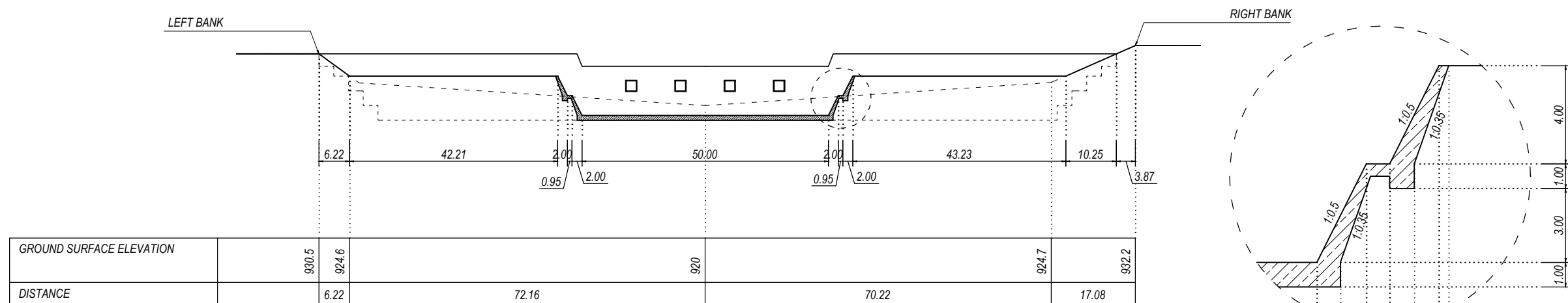
POTONGAN C - C SKALA 1:100
