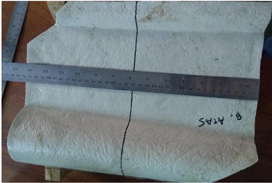
Proses pengujian analisis ukuran pada benda uji genteng komposit
