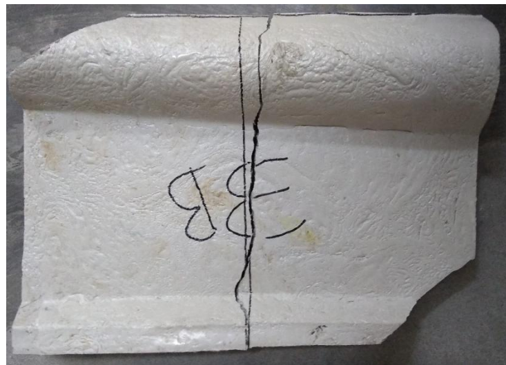
hasil pengujian beban lentur dengan rusak patah melintang
