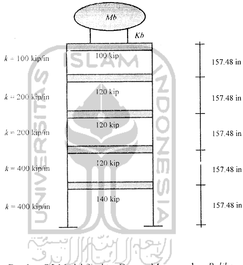
Gambar 5.2 Model Struktur Dengan Menggunakan Baliho
