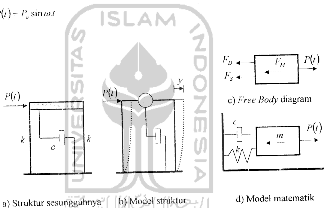
Gambar 3.1 Beban Dinamik Pada Struktur SDOF
