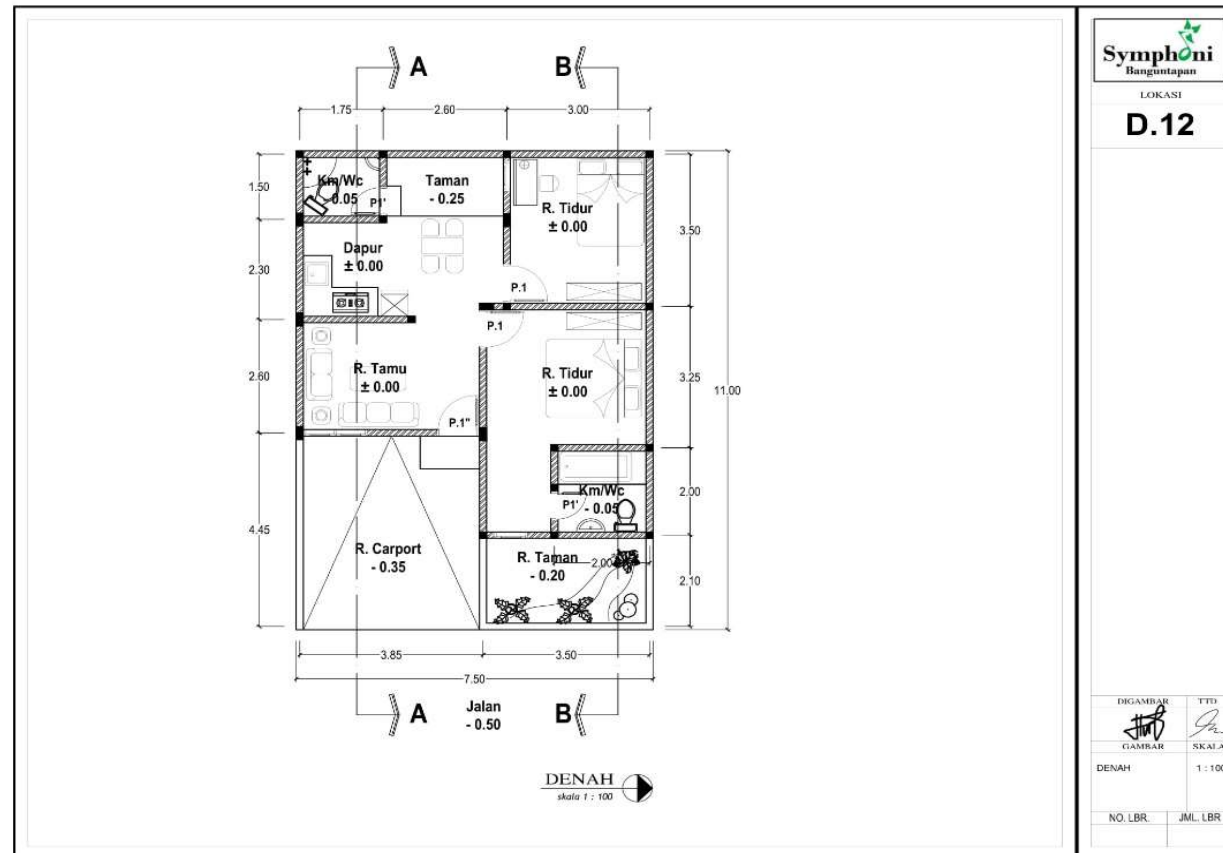
Gambar L-14 Denah Ruang Perumahan Symphoni
