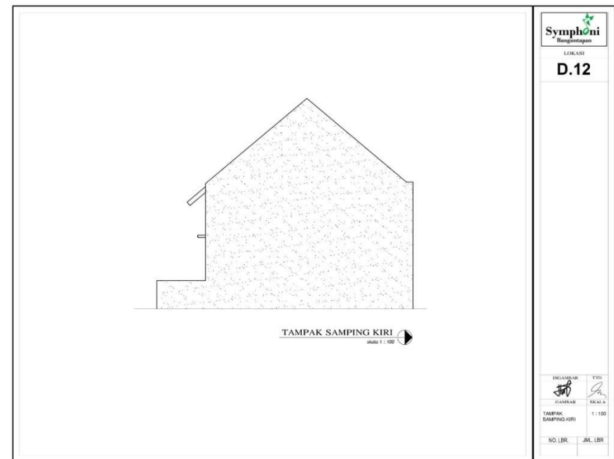
Gambar L-15.2 Tampak Samping Kiri
