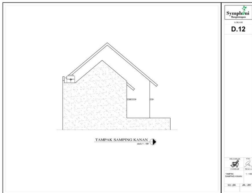
Gambar L-15.1 Tampak Samping Kanan
