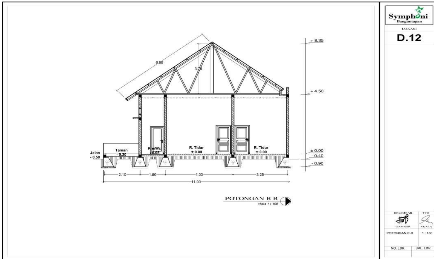
Gambar L-15.4 Potongan B-B
