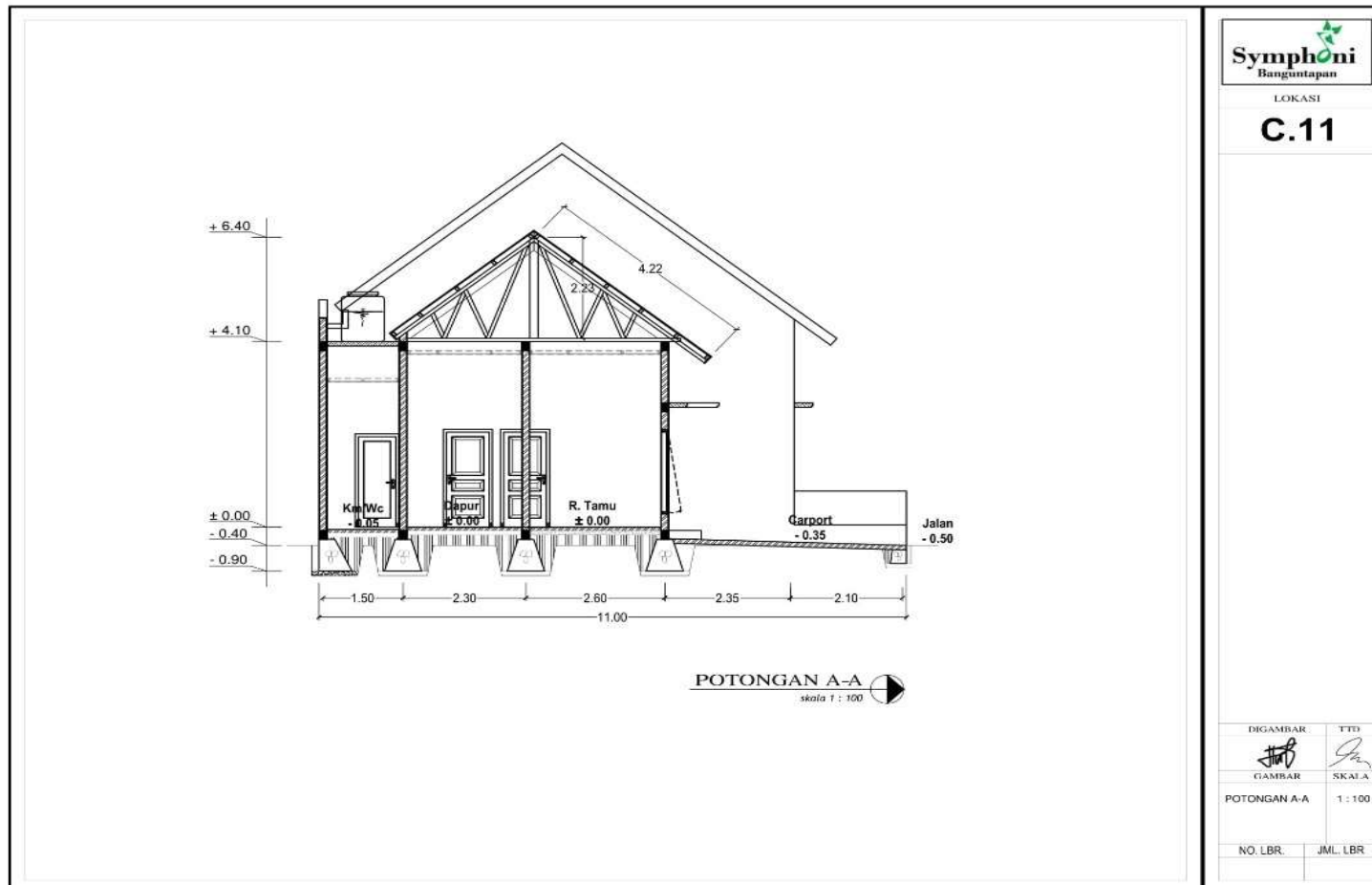
Gambar L-15.3 Potongan A-A
