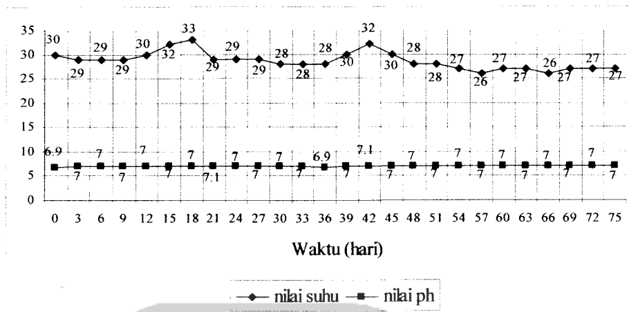
Gambar 4.6 Hubungan pH dan suhu pada reaktor II (85 : 10 : 5)
