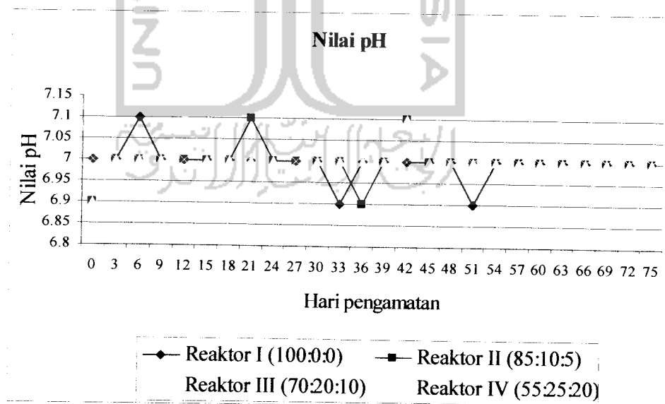
Gambar 4.2 Hasil pengukuran pH masing-masing reaktor
