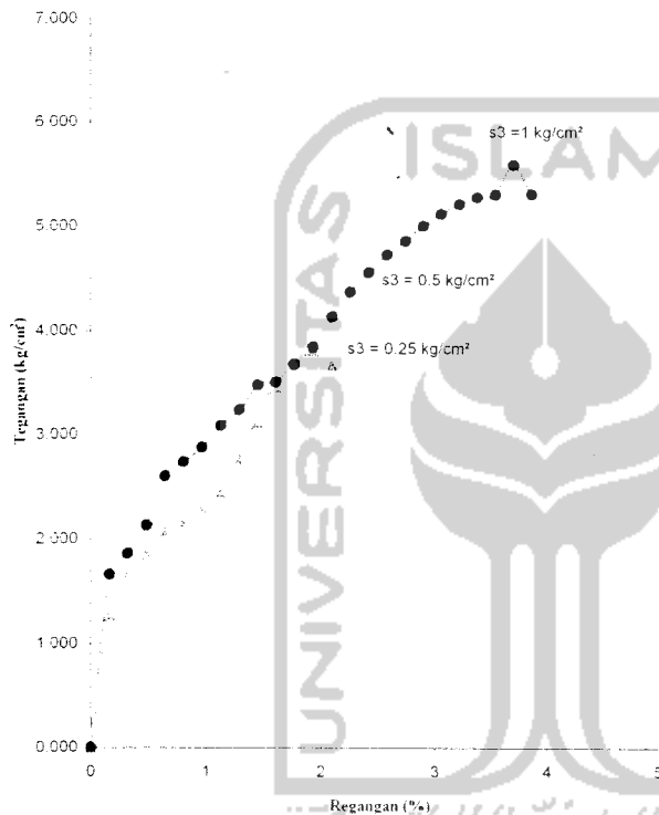
Grafik Tegangan-Regangan
