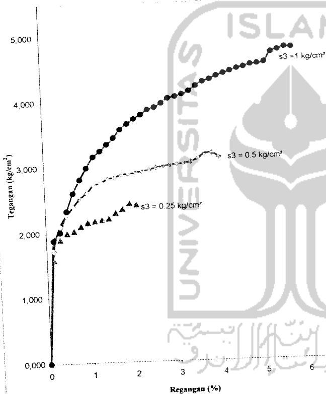
Grafik Tegangan-Regangan
