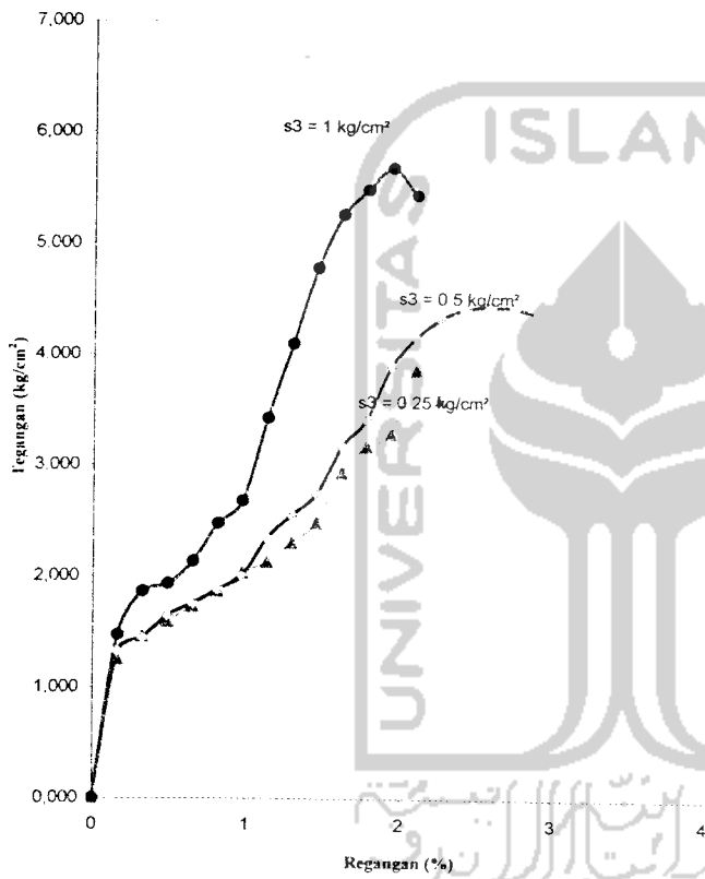
Grafik Tegangan-Regangan
