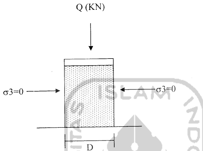
Gambar 3.5 Skema uji Tekan Bebas
