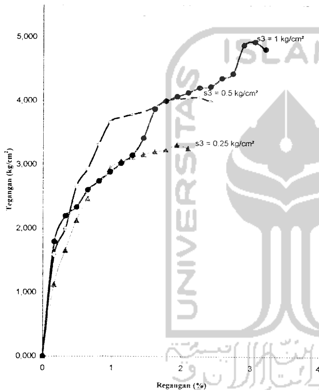
Grafik Tegangan-Regangan
