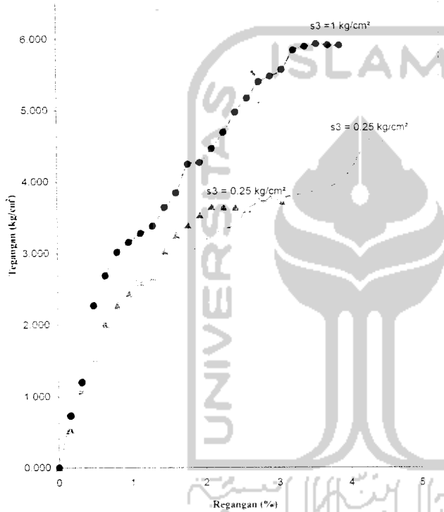
Grafik Tegangan-Regangan
