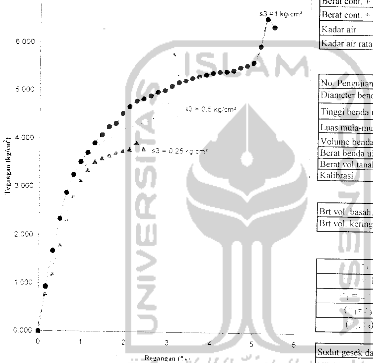
Grafik Tegangan-Regangan
