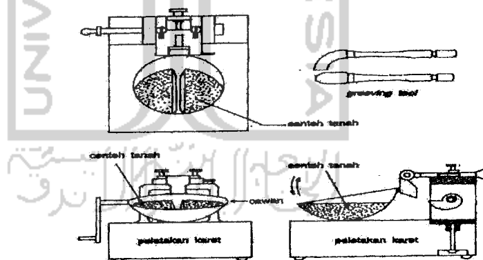
Gambar 3.4 Alat pengujian batas cair
