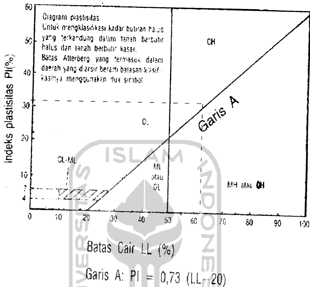
Gambar 6.2 Klasifikasi tanah berdasarkan sistem Unified
