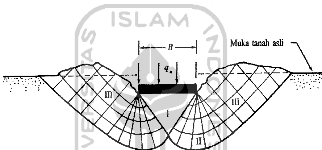
Gambar 3.5 Keruntuhan geser menyeluruh
