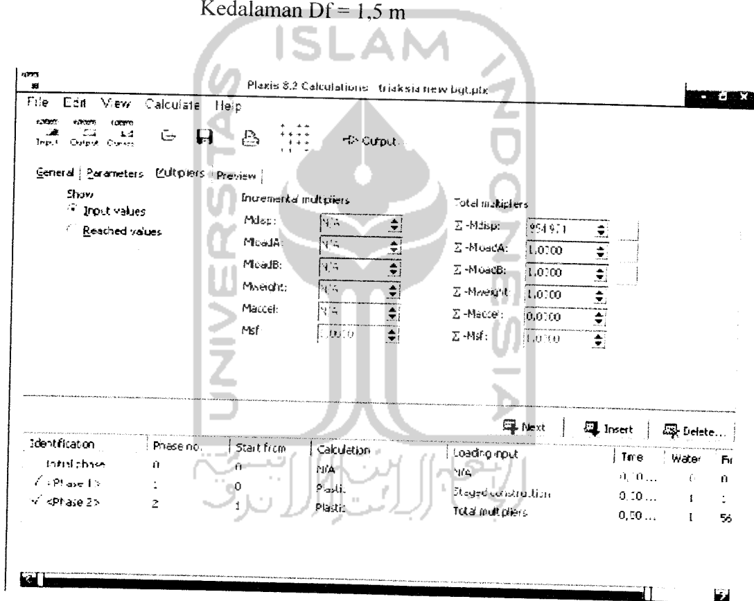
Gambar 5.17 Kalkulasi Program Plaxis dengan data yang dimasukkan data uji Triaksial dengan beban (P) 85,4971 ton.
