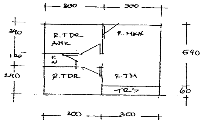
Gambar 47 Pengembangan Rangkaian Ruangan Model III
