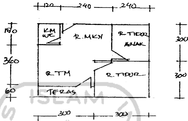
Gambar 45 Pengembangan Rangkaian Ruang Model I
