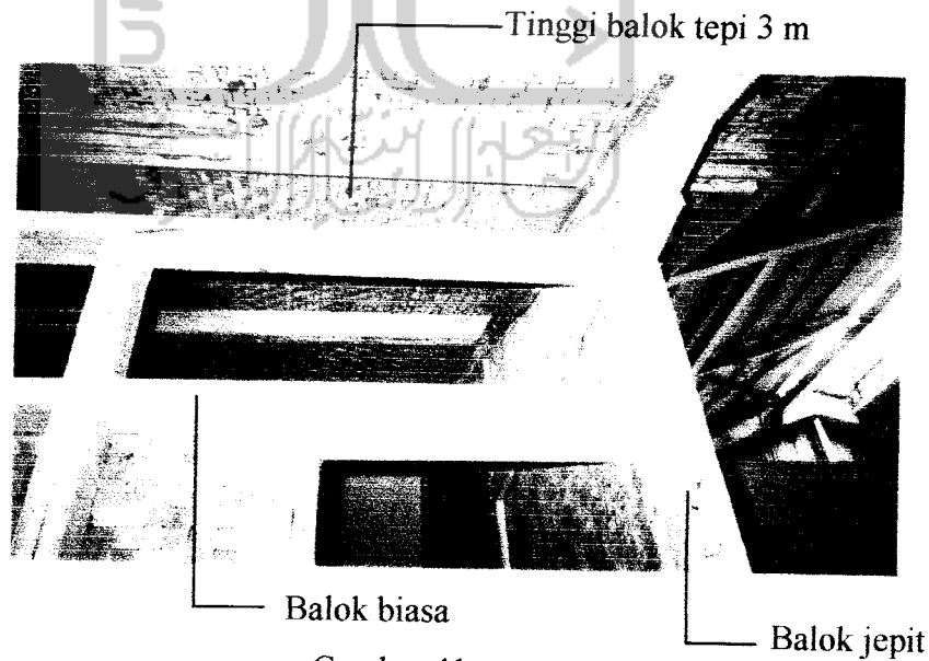
Gambar 41 Mok- Up Laminasi Bambu Sumber: Puskim Bandung
