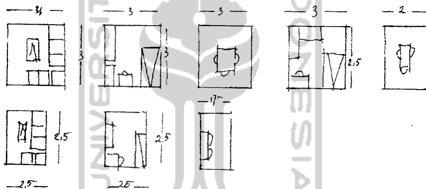
Gambar 5 Standar Ukuran Ruang (Tutu TW. Surowiyono, 2005)
