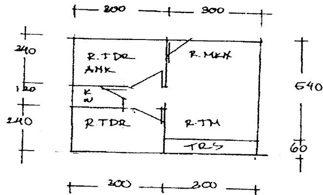
Gambar 20 Rangkaian Ruang Model Tiga Pengembangan
