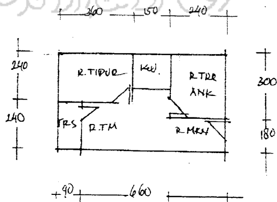
Gambar 49 Pengembangan Rangkaian Ruangan Model V
