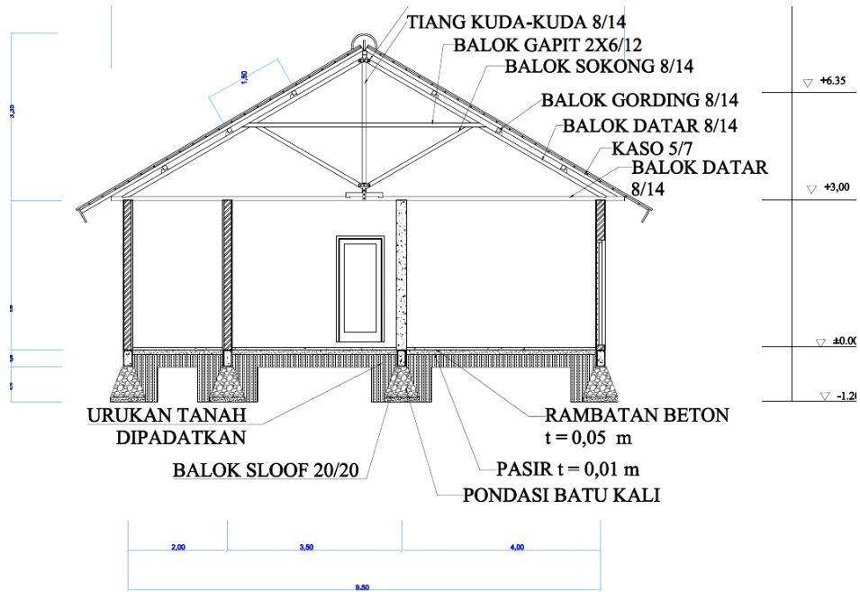
POTONGAN S-01
