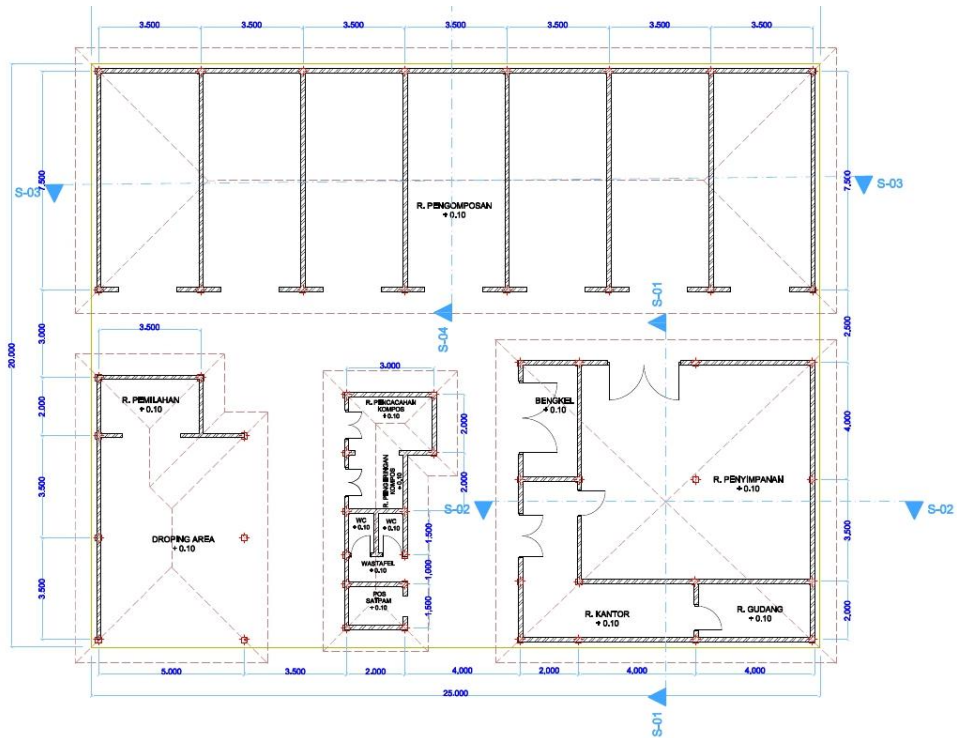
Gambar 5 Denah Perencanaan TPS dengan Konsep 3R
