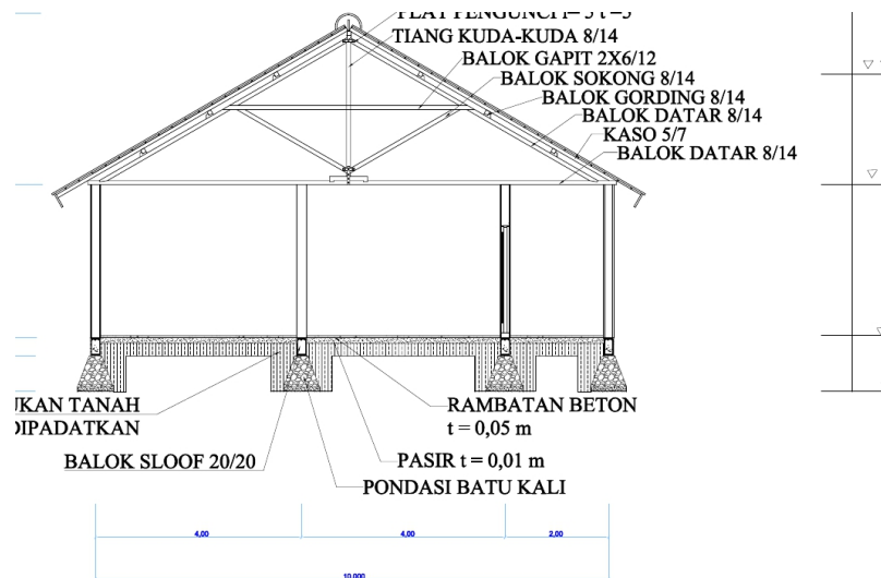
POTONGAN S-02
