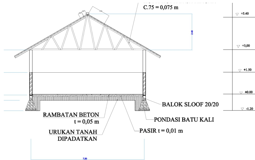
POTONGAN S-04
