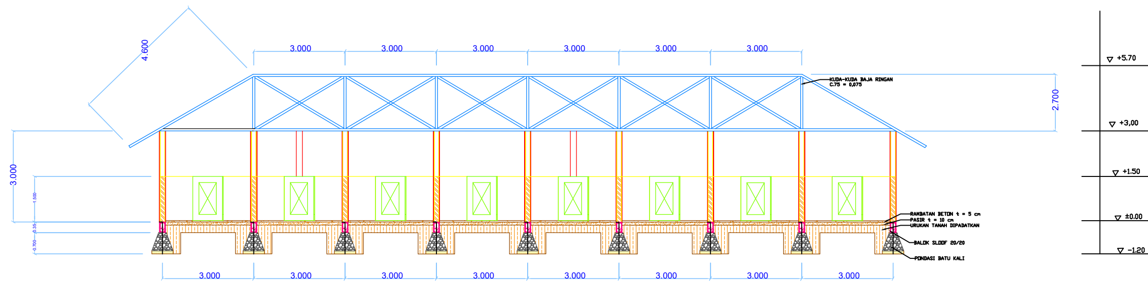
POTONGAN S-3
